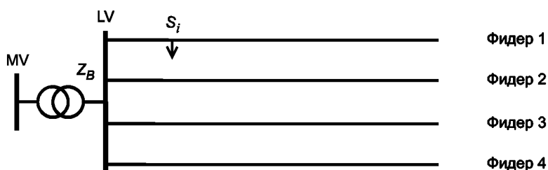
Рисунок Е.1 — Изучаемая низковольтная система
