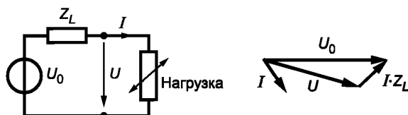
а) Эквивалентная схема
