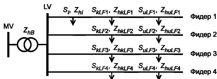
Рисунок F.1 — Изучаемая система
