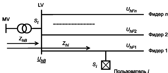
Рисунок 4 — Упрощенная схема общественной низковольтной системы для гармоник
