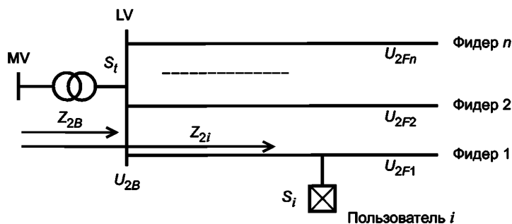
Рисунок 7 — Упрощенная схема общественной низковольтной системы при несимметрии
