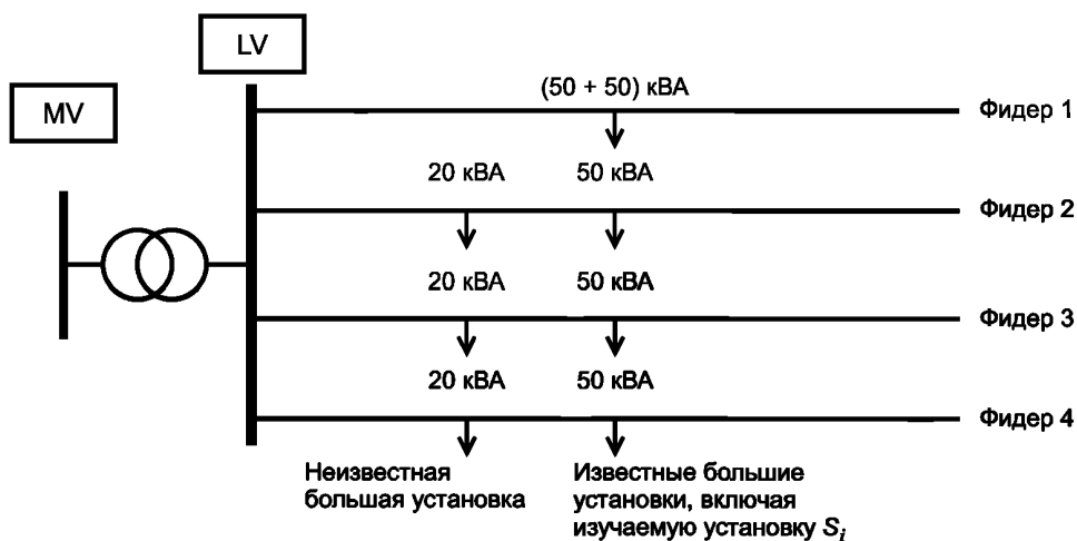
Рисунок F.2 — Данные о больших установках
