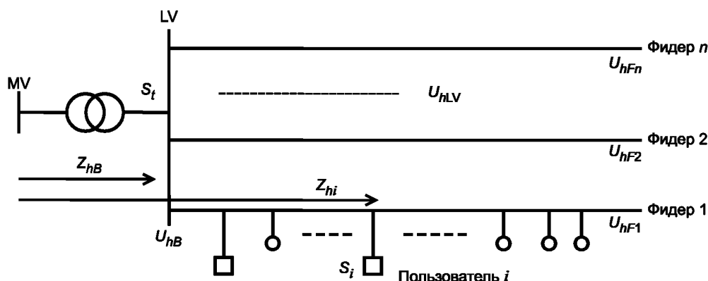
Рисунок С.1 — Схема общественной низковольтной системы
