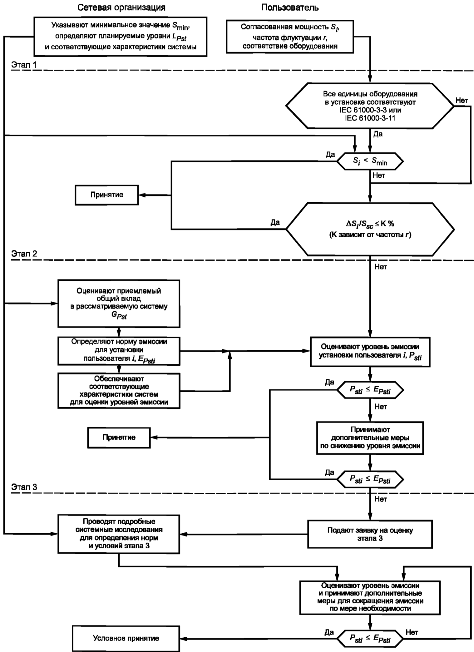
Рисунок 9 — Схема процедуры оценки колебаний напряжения
