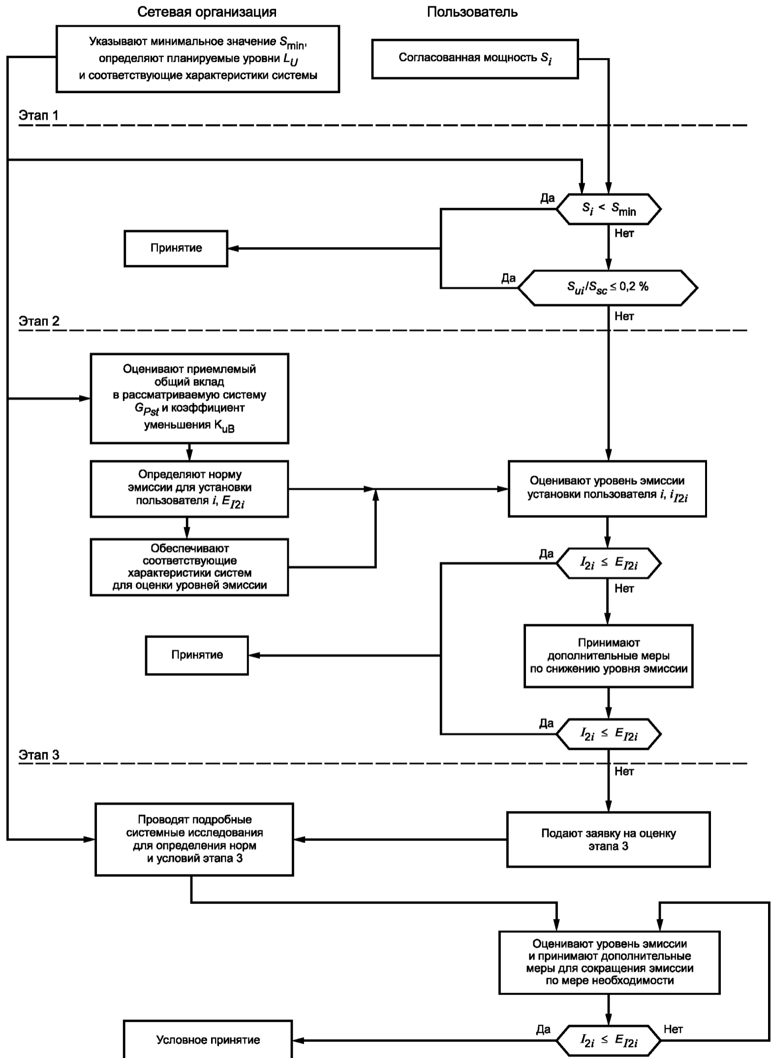
Рисунок 10 — Схема процедуры оценки несимметрии
