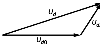
Рисунок 3 — Иллюстрация вектора эмиссии U_{di} и его вклада в измеряемый вектор помех U_d от установки в РОЕ
