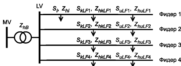
Рисунок E.2 — Компоненты большой установки
