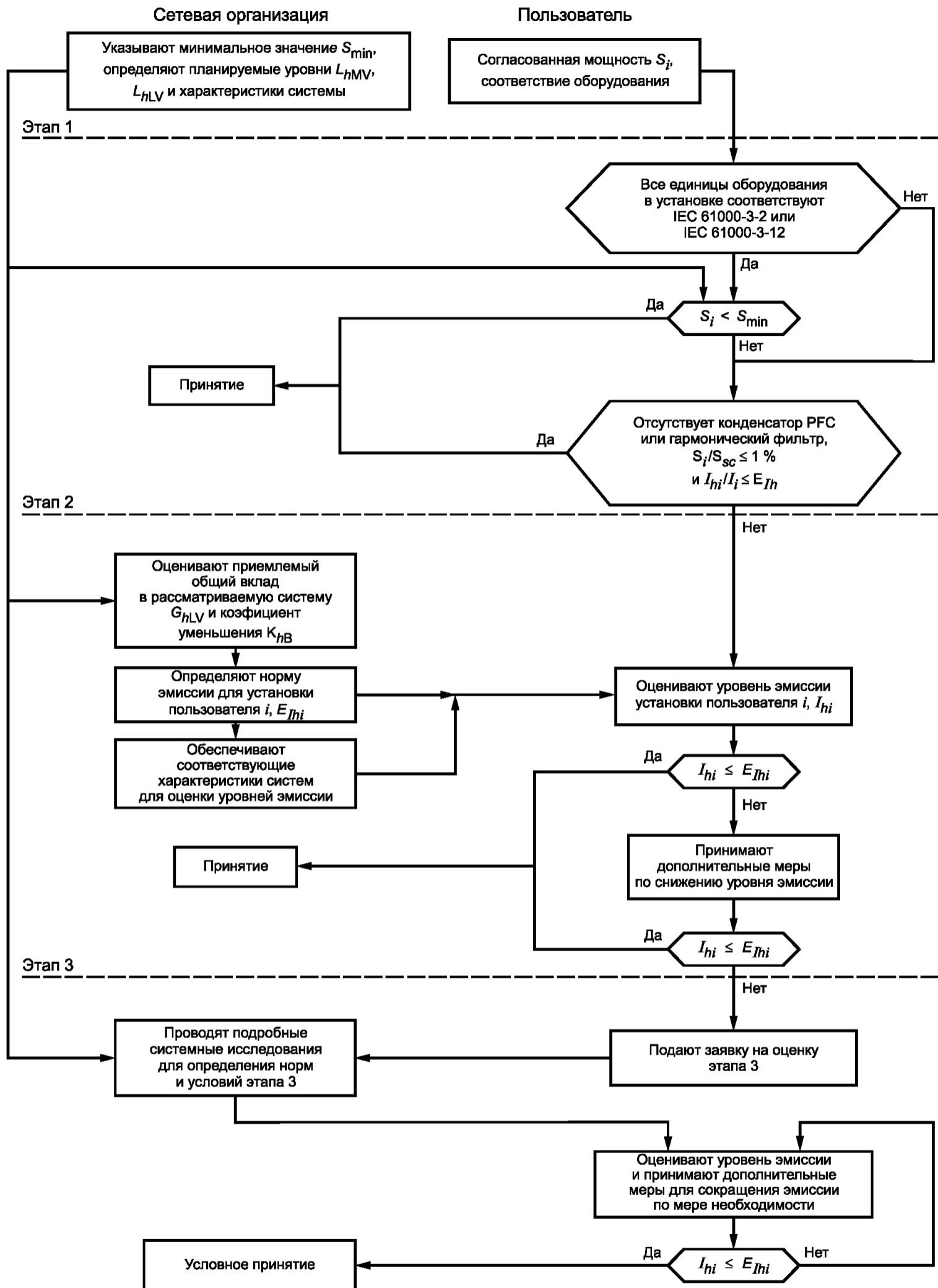
Рисунок 8 — Схема процедуры оценки гармоник
