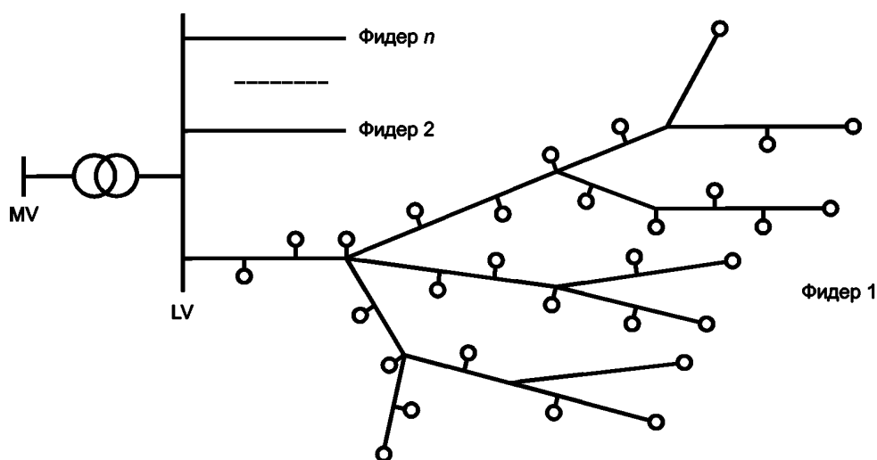
Рисунок D.1 — Общая схема общественной низковольтной системы
