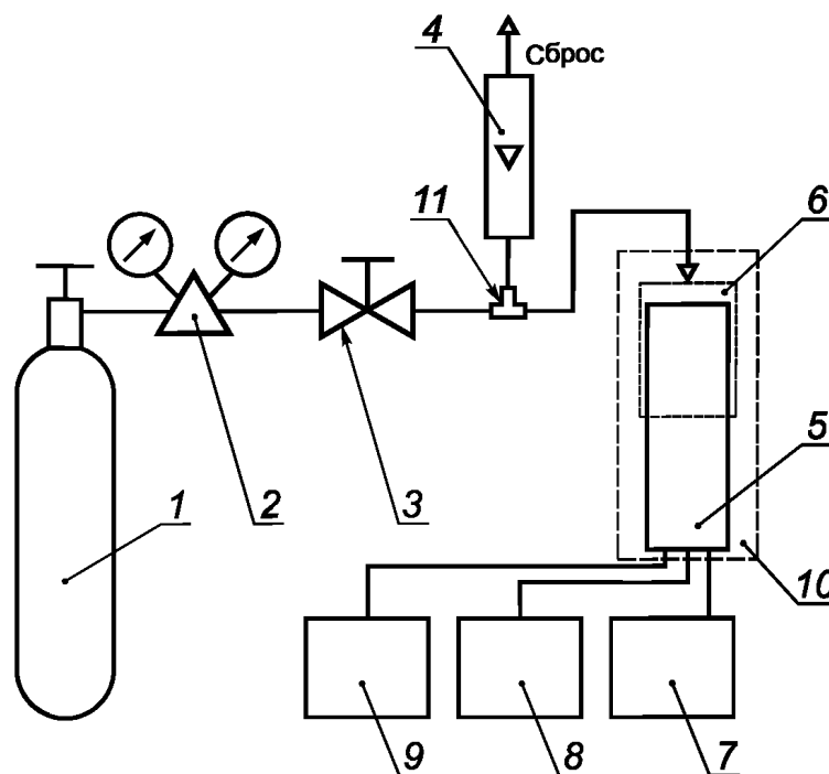
Рисунок А.1 — Схема подачи ГС на СИ с диффузионным отбором пробы при проведении поверки
