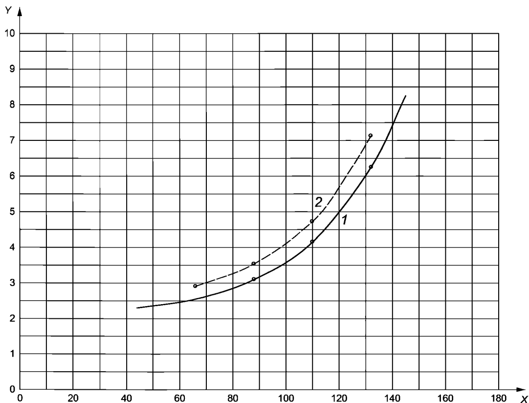
X — подача Q , \text{м}^3/\text{ч} при n = 2950 \text{ мин}^{-1} ; Y — кавитационный запас насоса NPSHR, м; 1 — вода; 2 — вязкая жидкость ( s = 0,90 , B = 12,0 )
