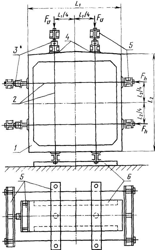
1—звено трубы; 2—металлические тяжи; 3—гидроомкраты; 4—слой цементно-песчаного раствора; 5—металлические тгаверсы; 6—опоры; F_v —вертикальная нагрузка; F_h —горизонтальная нагрузка
