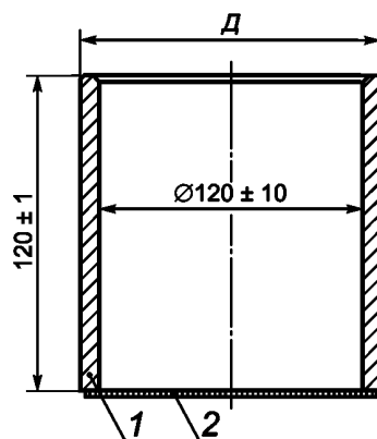
Рисунок 1 — Цилиндр
