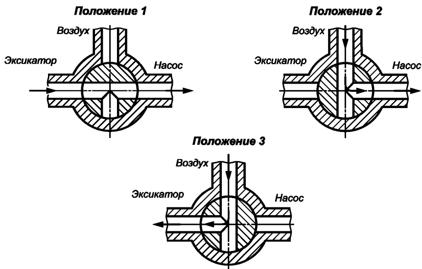
Рисунок 4 — Положения трехходового крана
