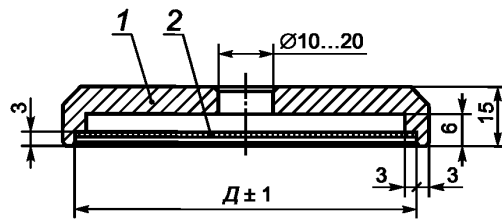
Рисунок 2 — Крышка
