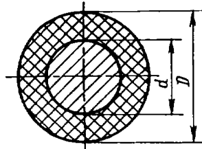
D —диаметр провода; d —диаметр проволоки
