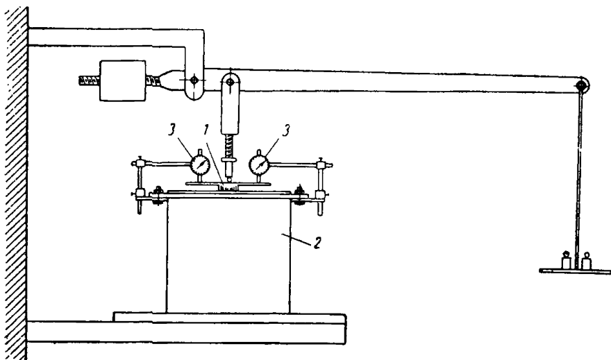
Рис. 11. Схема установки штампа и мессур:
