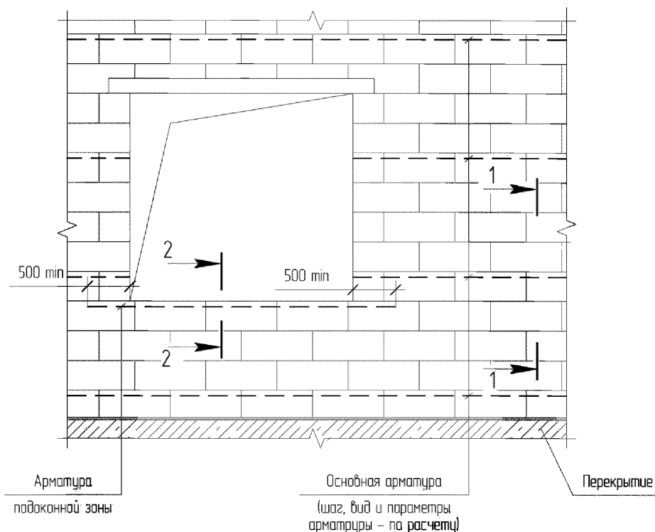
Рис. 3.5. Пример схемы армирования стен
