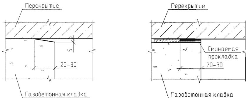
Рис. 4.2. Мероприятия, уменьшающие величину эксцентриситета нагрузки
