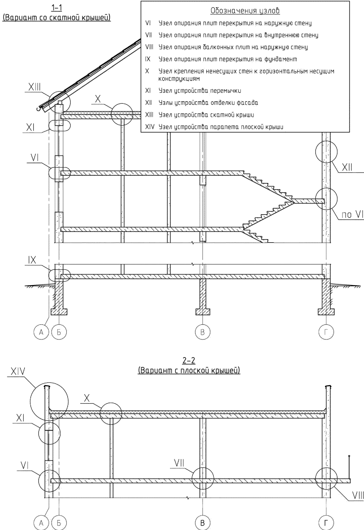
Рис. 4.8 Маркировочная схема узлов (разрезы 1-1 и 2-2)
