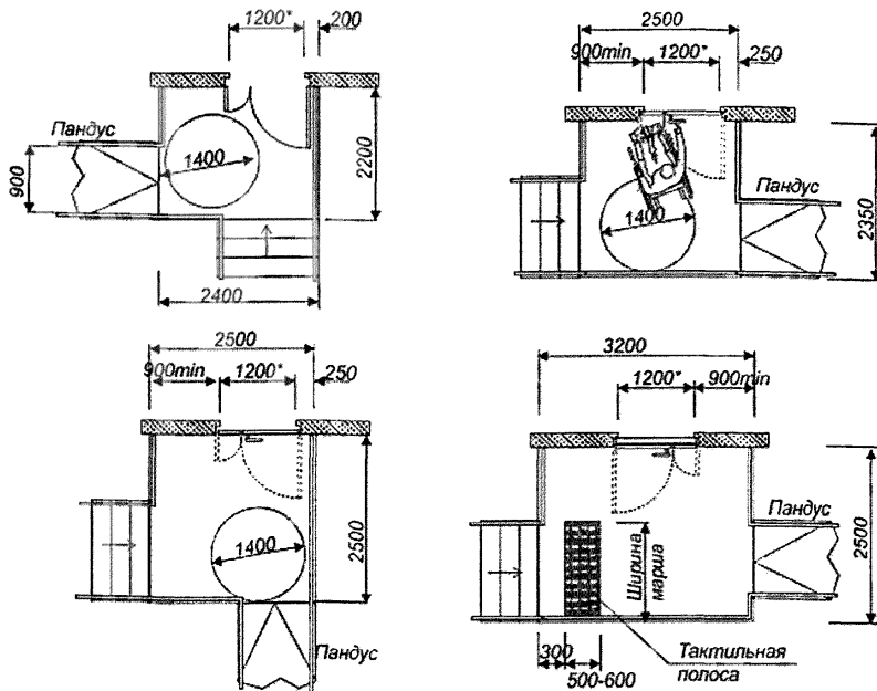
Рисунок В.19 - Площадки перед входами
