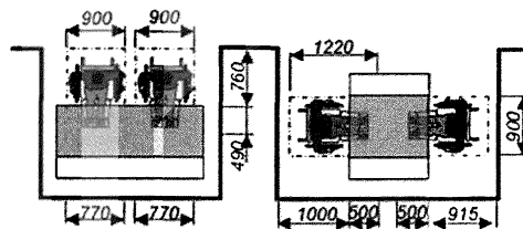
Рисунок Г.5 - Габариты у мест обслуживания
