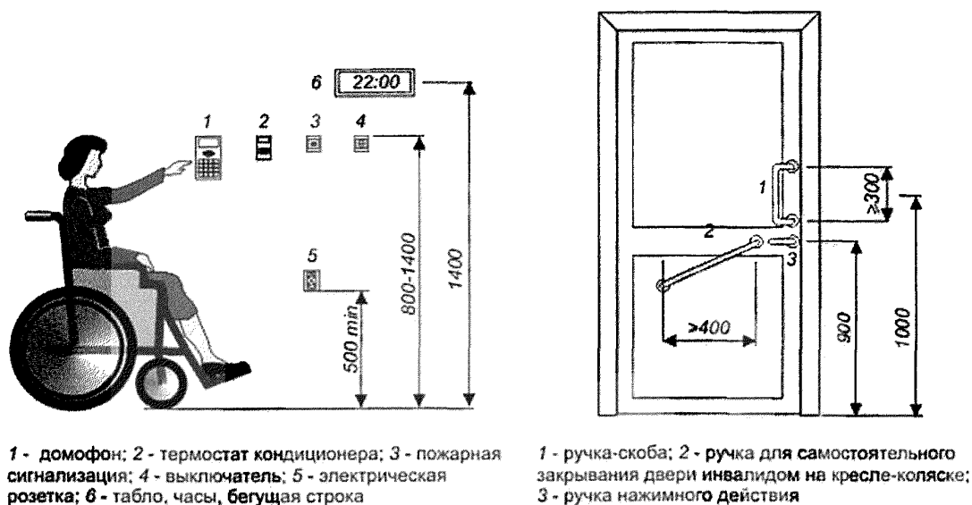
Рисунок Г.6 - Досиаемость оборудования
