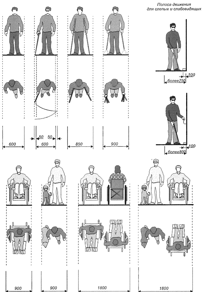
Рисунок В.11 - Габариты полосы движения
