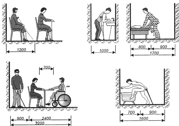
Рисунок Г.4 - Параметры функциональных зон
