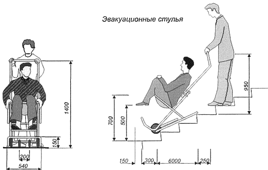
Рисунок В.34 - Автономные транспортные устройства
