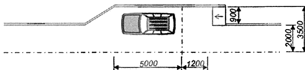
Рисунок В.9 - Стоянки автомобилей
