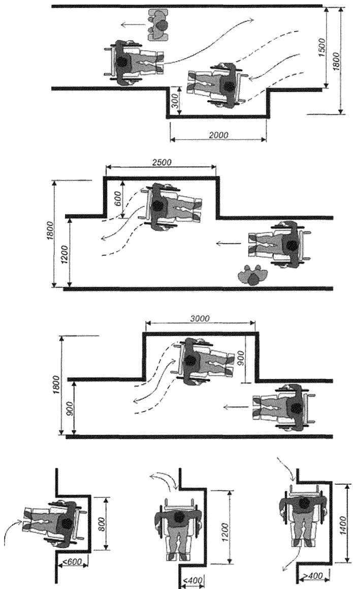
Рисунок В.15 - Ниши в коридорах
