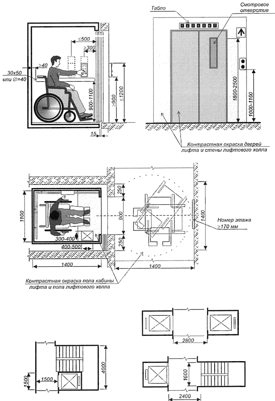
Рисунок В.30 - Оборудование лифтов
