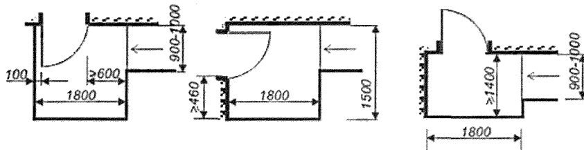
Конечные площадки
