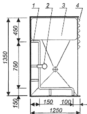
Непроходная кабина
