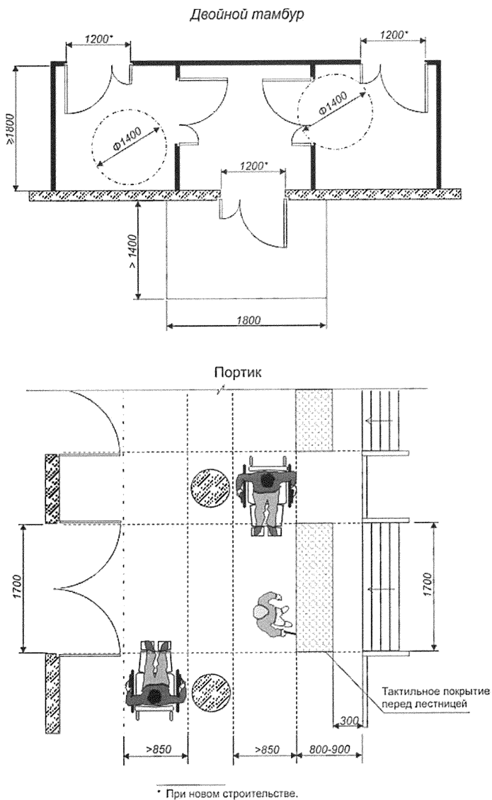
Рисунок В.21 - Площадки перед тамбуром и портиком
