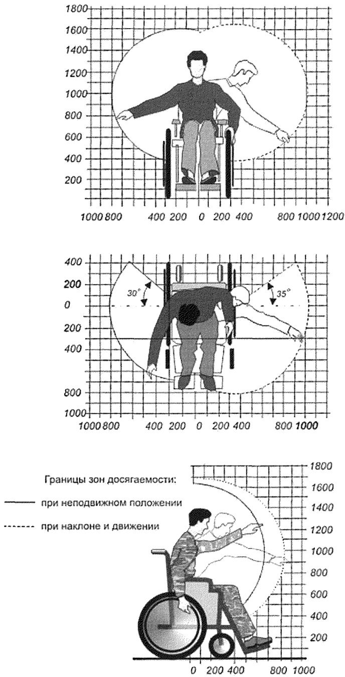
Рисунок Г.1 - Зоны досягаемости инвалидов на кресле-коляске
