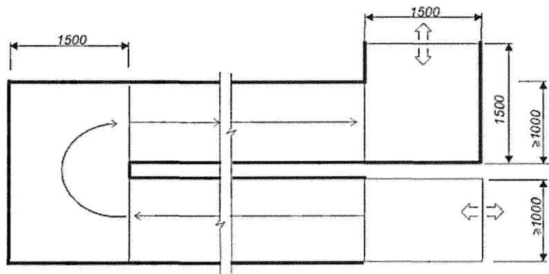
Промежуточные площадки
