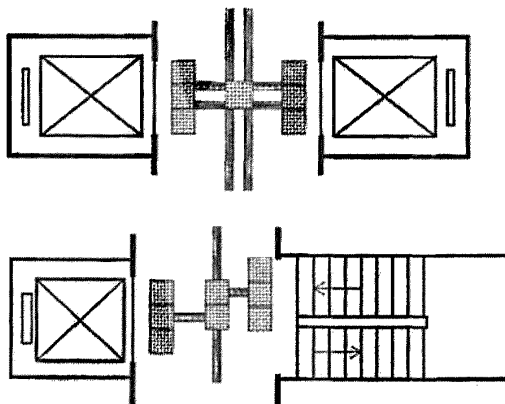
Рисунок Г.18 - Тактильно-контрастные указатели
