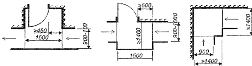
Конечные площадки
