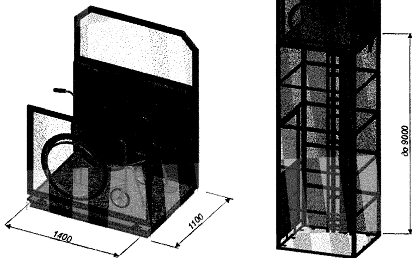
Рисунок В.33 - Параметры вертикальных подъемников
