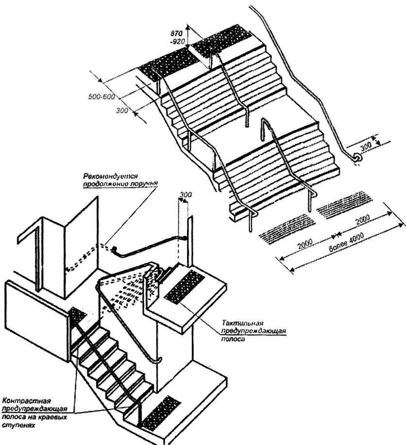
Рисунок В.24 - Параметры лестниц
