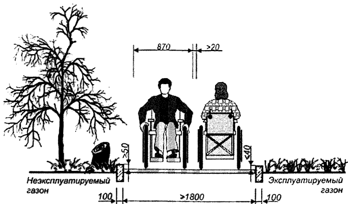
Рисунок В.7 - Организация путей движения на участке
