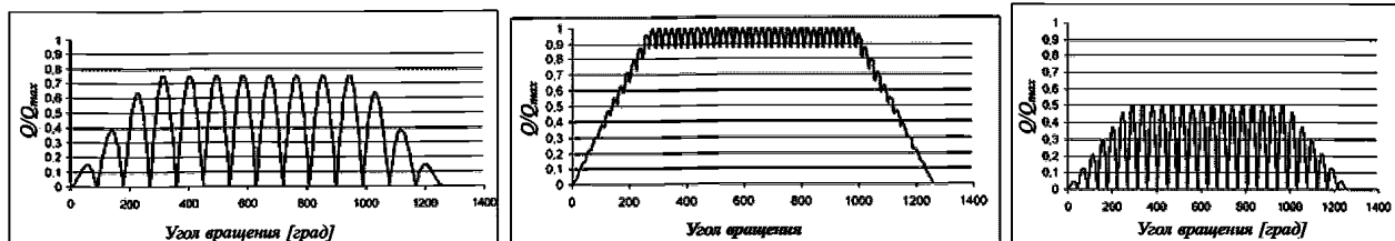
Рис. 10.7.5.3.3 Процесс изменения ледового момента сопротивления вращению четырехлопастного гребного винта для последовательности 90° и 135° одиночного взаимодействия и 45° двойного взаимодействия гребного винта со льдом
