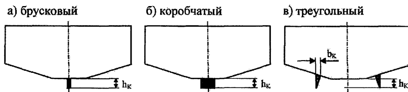
г) возможное расположение фальшекилей по ширине судна
