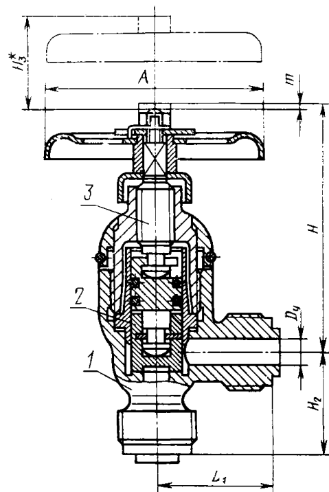
1—корпус; 2—тарелка; 3—шпindelь Черт. 3
