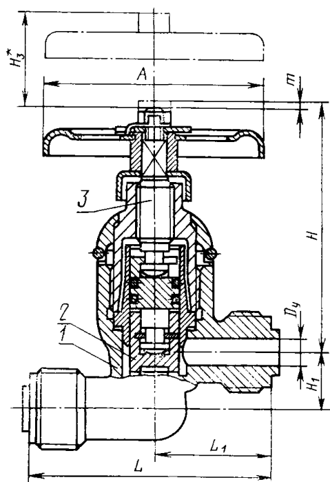
1—корпус; 2—тарелка; 3—шпindelь Черт. 1
