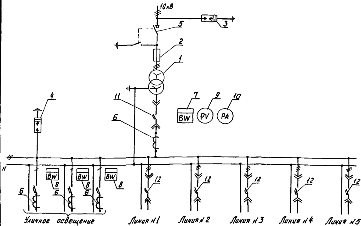
СХЕМА ЭЛЕКТРИЧЕСКИХ СОЕДИНЕНИЙ ПОДСТАНЦИИ
