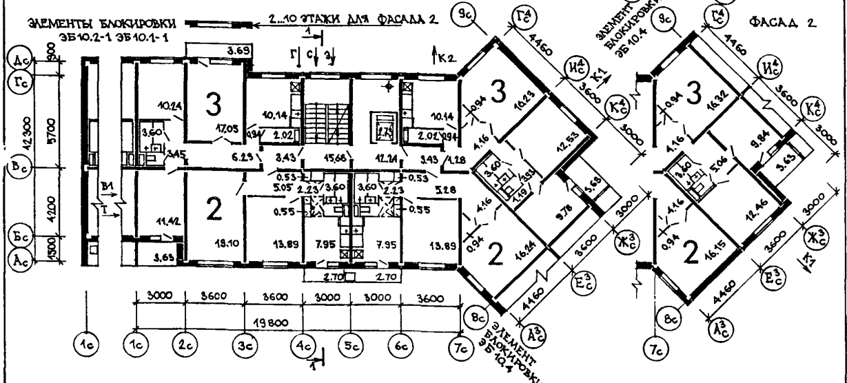
ЭКСПЛИКАЦИЯ КВАРТИР
