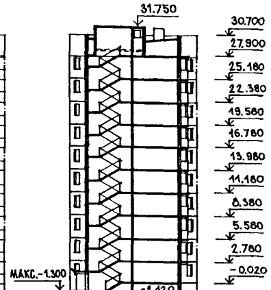
РАЗРЕЗ 1-1
