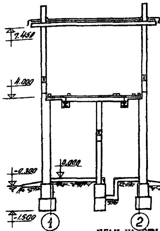
РАЗРЕЗ I-I
