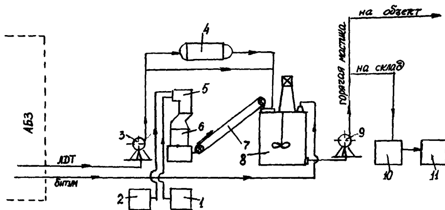
Рис.1. Технологическая схема приготовления полимерно-битумной мастики на АБЗ I - склад для ЛДТ; 2 - склад для асбеста; 3,9-насосы; 4 - теплообменник; 5 - пневматический нож (дробилка); 6 - сушилка; 7 - транспортер; 8 - котел-смеситель; 10 - брикетные формы; 11 - склад для хранения готовой мастики
