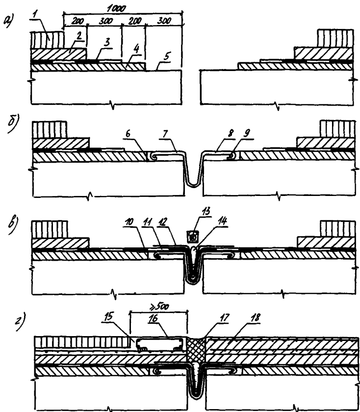
Рис.13. Реконструкция швов заполненного типа: а-ступенчатая вырубка слоев дорожной одежды; б-установка металлического компенсатора; в-устройство гидроизоляции; г-заполнение зазора и бетонирование покрытия; 1-асфальтобетонное покрытие; 2-защитный слой; 3-гидроизоляция; 4-выравнивающий слой; 5-поверхность балок; 6-полимерраствор; 7-металлический компенсатор; 8-анкерные полосы компенсатора; 9-продольный стержень; 10-утяжеленный рулонный гидроизоляционный материал; 11-гидроизоляция; 12-полиэтиленовая пленка; 13-опалубочная доска (рейка); 14-пористый заполнитель; 15-бетонный прилив; 16-арматурный каркас; 17-мастика заполнения; 18-бетонное покрытие
