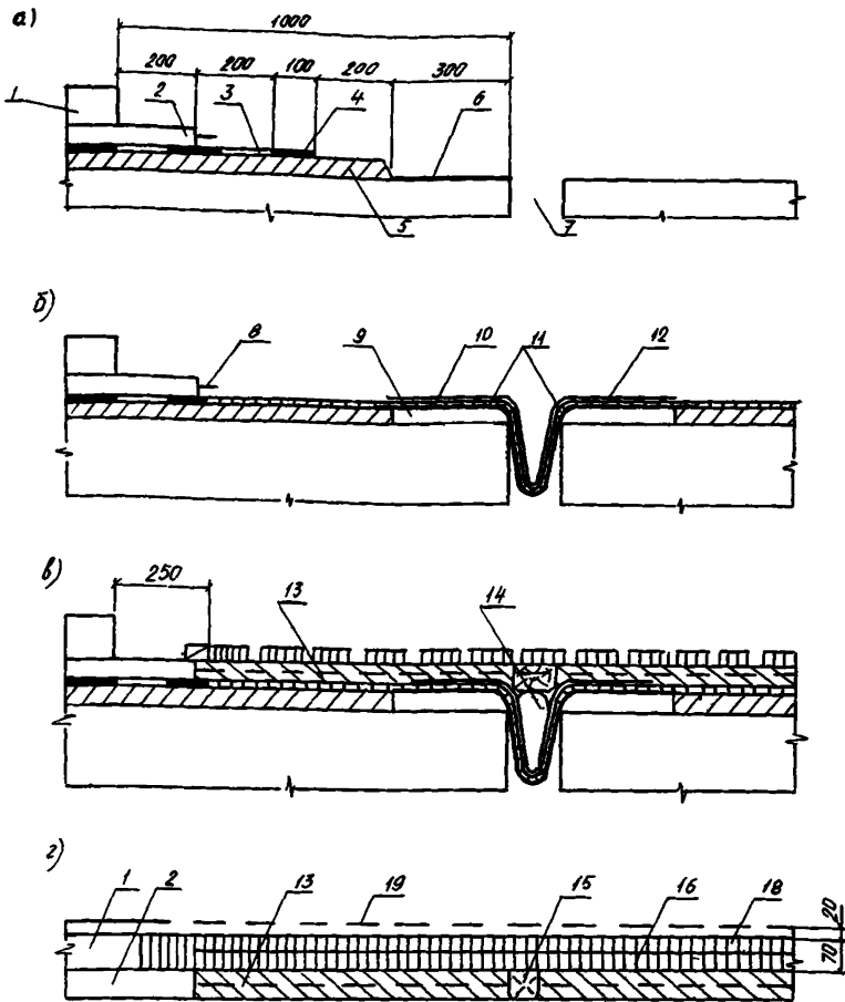
Рис.10. Реконструкция шва закрытого типа:
