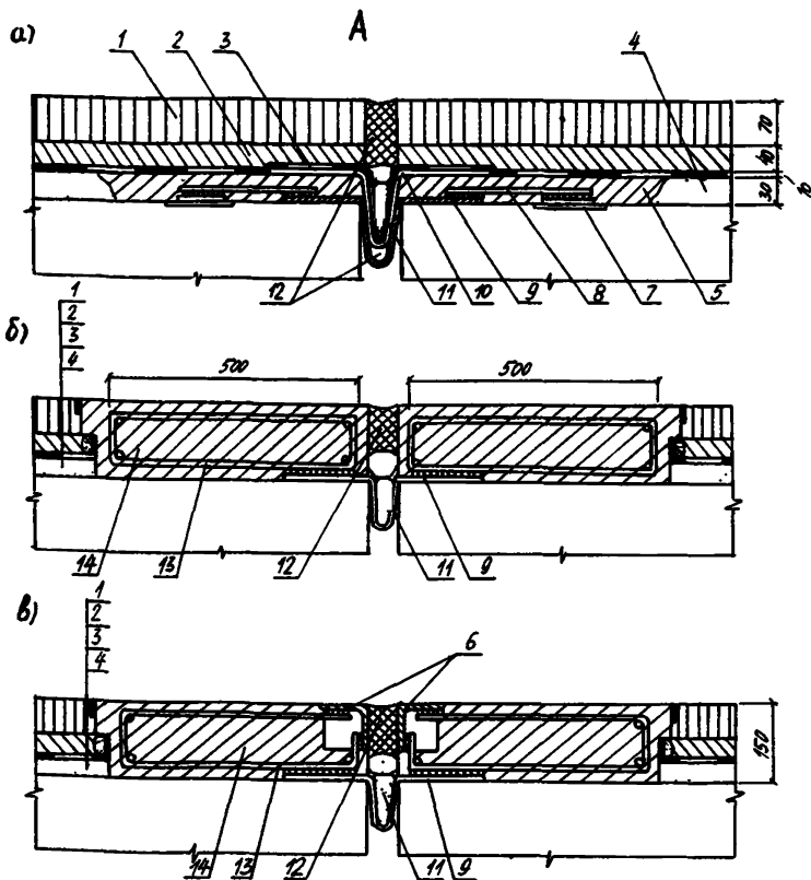
Рис.2. Конструкции деформационных швов заполненного типа
