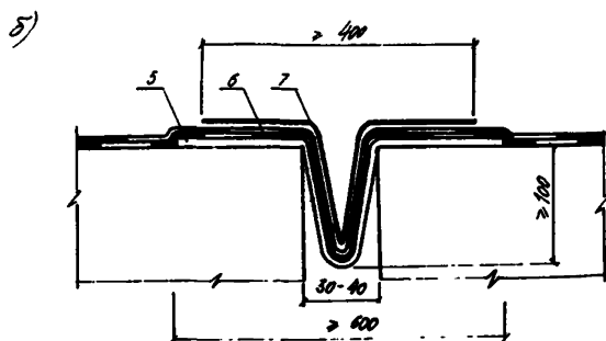
Рис.3. Металлический (а) и неметаллический (б) компенсаторы деформационных швов:
