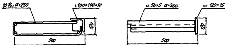
Рис. 6. Сечение окантований деформационных швов
