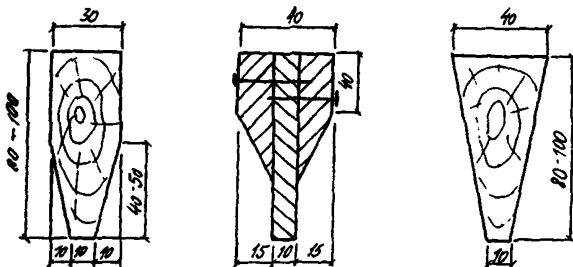
Рис. 5. Сечение уплотнителей для деформационных швов
