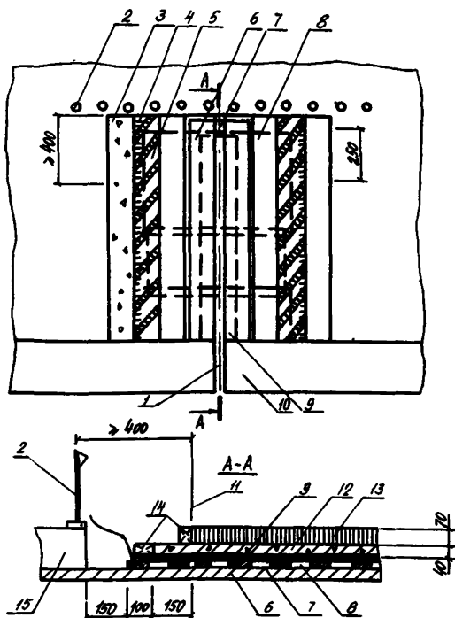
Рис. II. Схема вырубki слоев дорожно ю одежды и их восстановления при реконструкции швов закрытого типа
