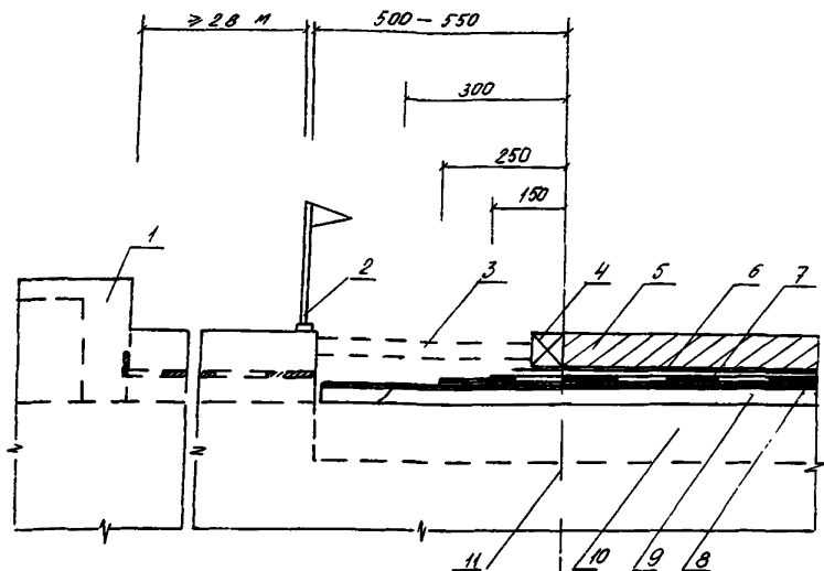
Рис.15. Расположение слоев ездового полотна при восстановлении конструкции швов заполненного типа с бетонным приливом:
