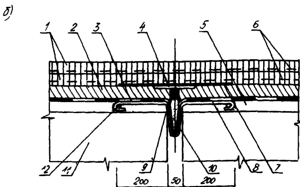
Рис. I. Конструкции деформационных швов закрытого типа: а - с непрерывным асфальтобетонным покрытием; б - с армированным покрытием; 1-асфальтобетонное покрытие; 2-защитный слой; 3-гидроизоляция; 4-металлическая пластина, перекрывающая зазор ( \delta = 0,10 втплена в защитный слой); 5-выравнивающий слой; 6-армирующие сетки; 7-отделяющая прокладка; 8-компенсатор; 9-битумная мастика; 10-пористый наполнитель; 11-балка; 12-ядерный стержень; 13-уплотнитель
