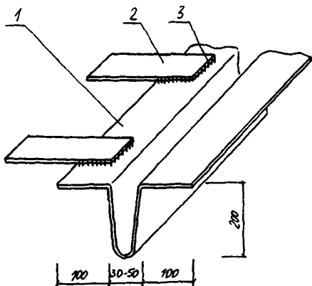
Рис. 4. Металлический компенсатор для деформационных швов заполненного типа:
