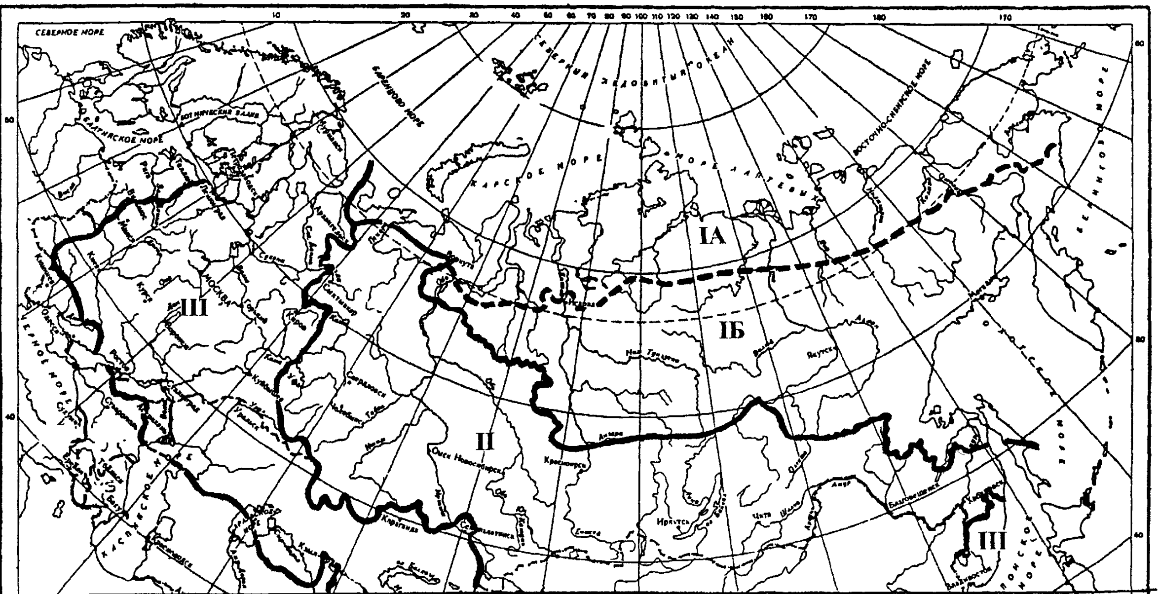
Схема районирования территории Российской Федерации по климатическим регионам
