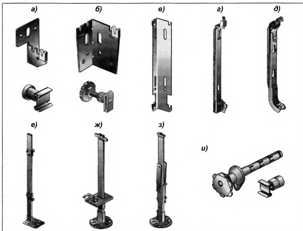
Рис. 1.3. Кронштейны для настенной и напольной установки радиаторов «RADIK»: а) кронштейн настенный одинарный простой (расстояние от радиатора до стены D=40 мм); б) кронштейн настенный угловой (D=36 мм и 54 мм); в) кронштейн настенный двойной (D=36 мм и 43 мм); г) кронштейн компактный (D=43 мм); д) кронштейн компактный ПЛЮС (D=30 мм); е) кронштейн-подставка внешний (расстояние от радиатора до пола T=170-270 мм); ж) кронштейн-подставка внешний для типов 20, 21 (T=100-200 мм); з) кронштейн-подставка внутренний для типов 11, 22, 33 (T=140-200 мм); и) кронштейн-шуруп (D=35-100 мм)
