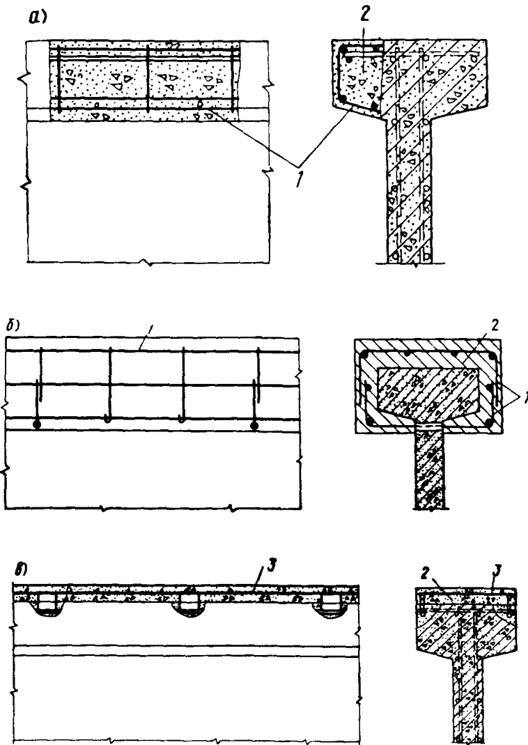
Рис. 6. Усиление сжатой полки балок a — заделка скоса в свесе полки; б — трехстороннее наращивание верхней полки; в — наращивание полки по верху; 1 — дополнительный каркас; 2 — заделка бетоном на мелком щебне; 3 — каркас набетонки, связанный с верхней арматурой балки
