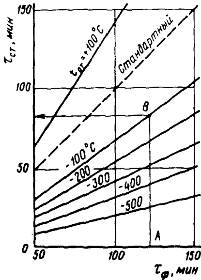
Рис. 1. График приведения фактического температурного режима к стандартному \tau_{ст} — длительность стандартного пожара; \tau_{ф} — длительность фактического пожара; t_{от} — разница в максимальной температуре фактического t_{ф} и стандартного t_{ст} пожаров ( t_{от} = t_{ф} - t_{ст} )
