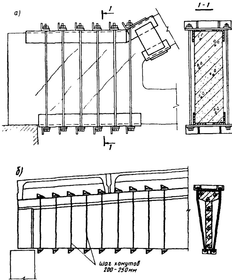
Рис. 8. Усиление опорной части конструкций наружными напрягаемыми хомутами а – усиление опорного узла фермы; б – усиление опорной части балки
