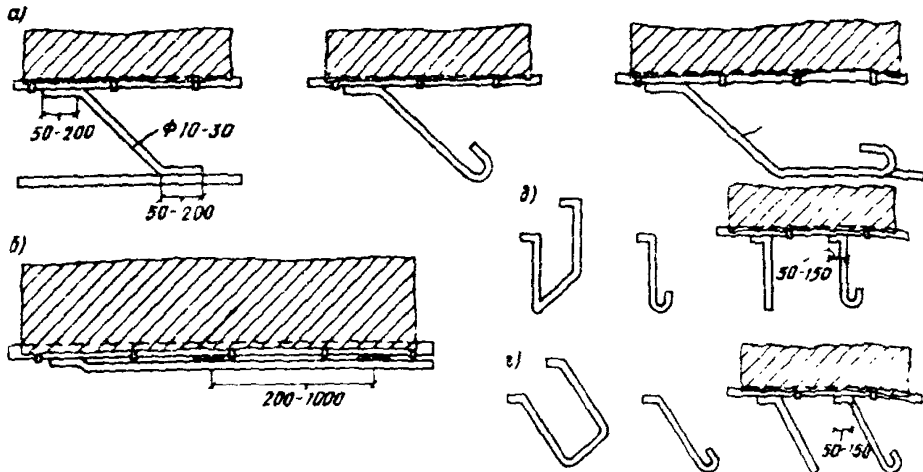
Рис. 2. Детали приварки арматуры усиления по методу И.М. Литвинова а — стобы и "утки" ( \phi 10-30 ); б — коротышки ( \phi 10-40 ); в — прямые ла- муты ( \phi 10-25 ); г — косые хомуты ( \phi 10-25 )
