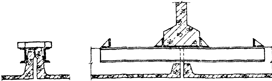
Рис. 14. Усиление ребристых плит перекрытий двухконсольными балочными системами
