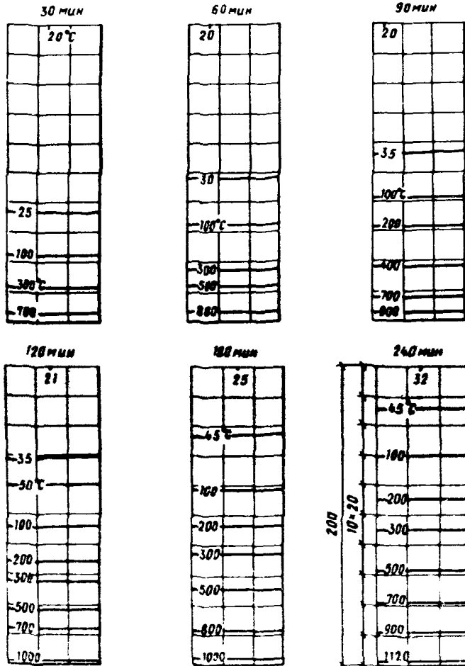
Рис. 15. Плита из легкого бетона, толщина 200 мм, нагрев с одной стороны
