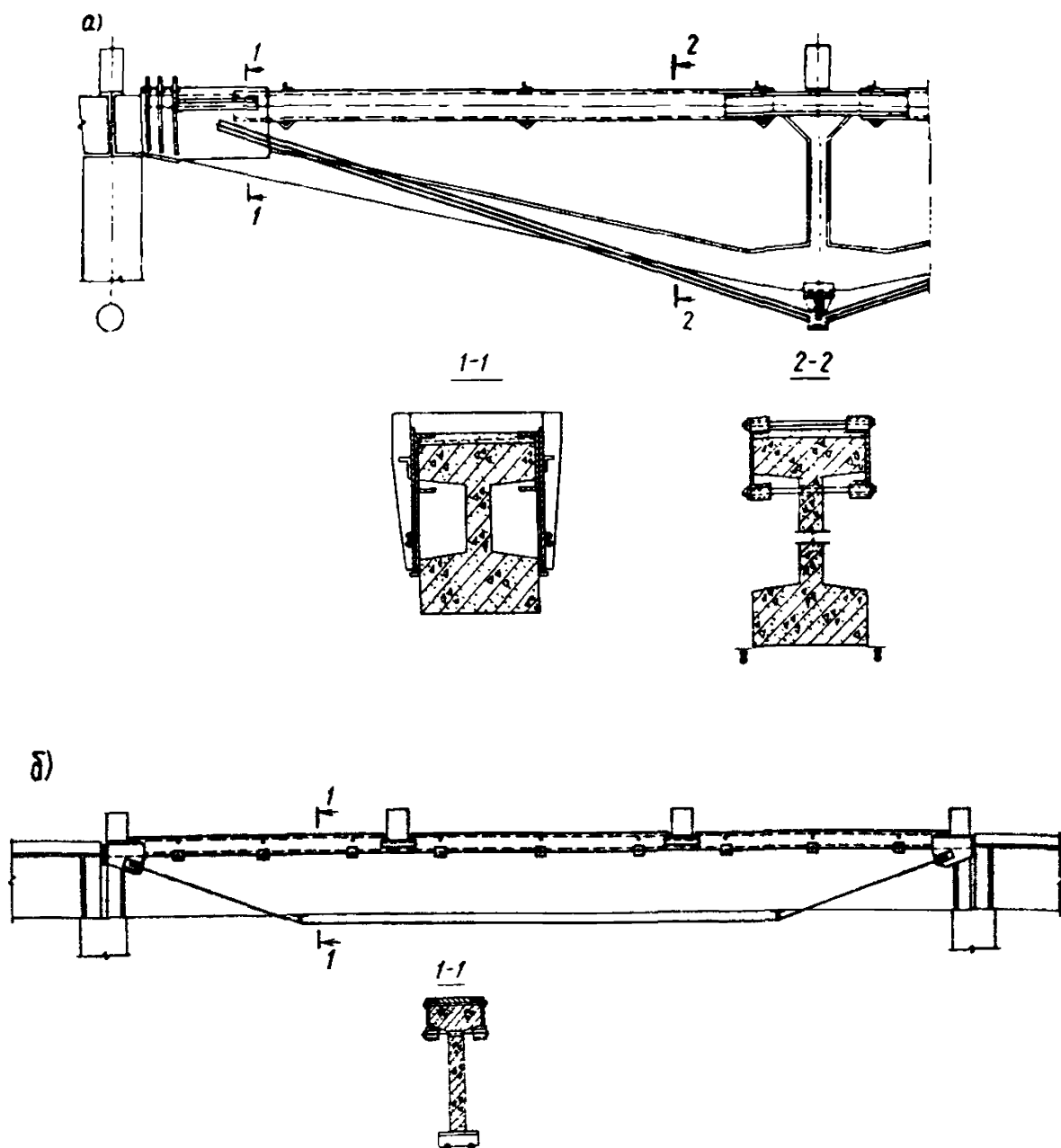
Рис. 11. Усиление растянутой и сжатой зоны балки а – затяжка треугольного очертания; б – шпренгельная затяжка
