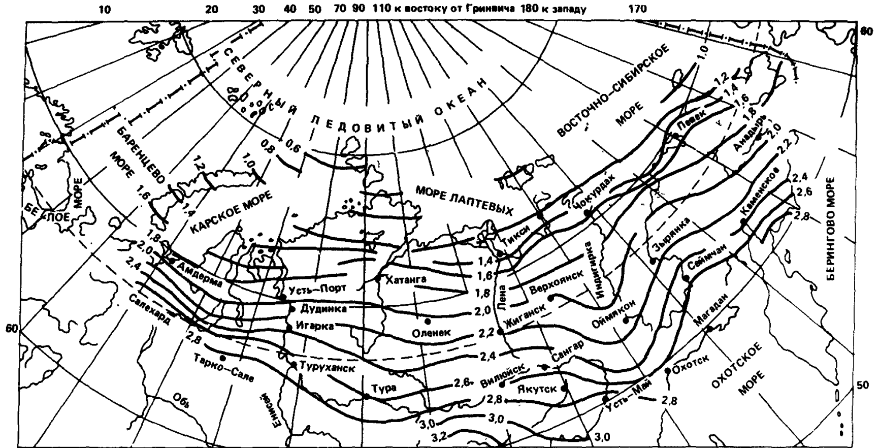
Рис. 21. Изолинии глубин сезонного протаивания песчаных грунтов, подстилаемых глинистыми
