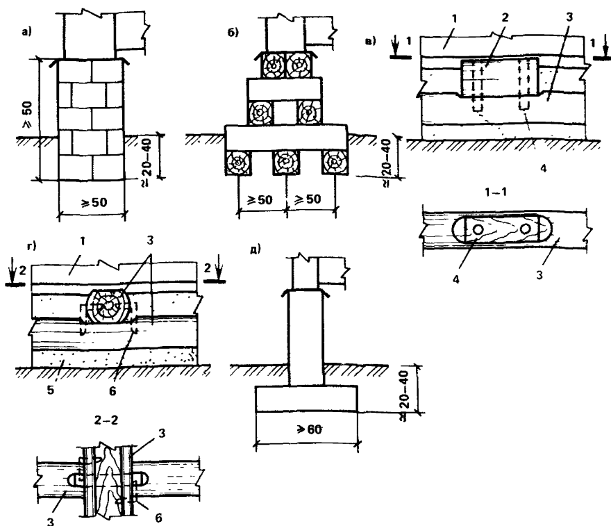
Рис. 1. Малозаглубленные фундаменты зданий из блок-контейнеров и крупнопанельных а, д – столбчатые из бетонных (железобетонных) элементов или кирпича; б – в виде деревянной клетки; в, г – из перекрестных деревянных балок; 1 – здание; 2 – подкладка; 3 – балка; 4 – нагели; 5 – песчаная подсыпка толщиной не менее 10 см; 6 – стальные скобы
