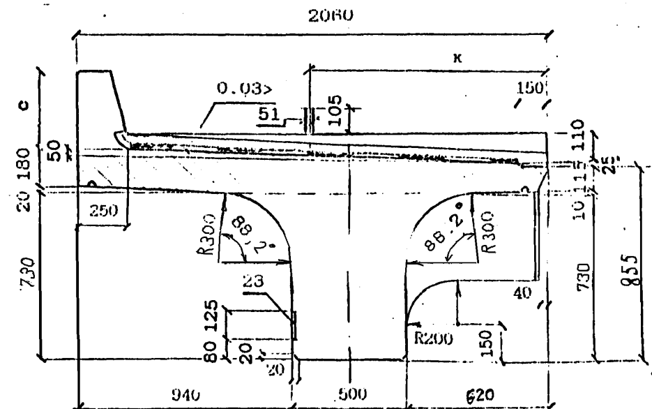
1 - 1 1:20
