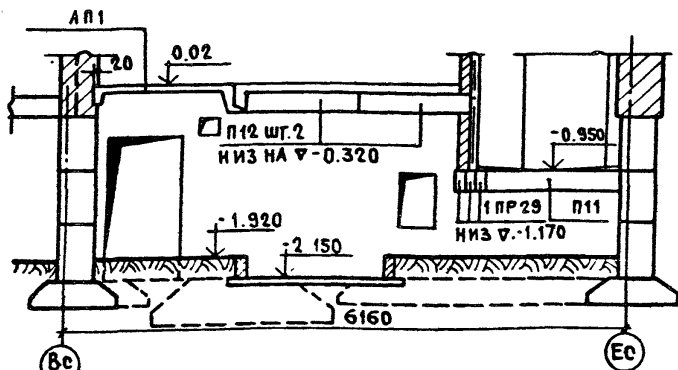
РАЗРЕЗ 7-7
