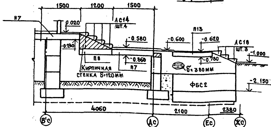
РАЗРЕЗ 8-8
