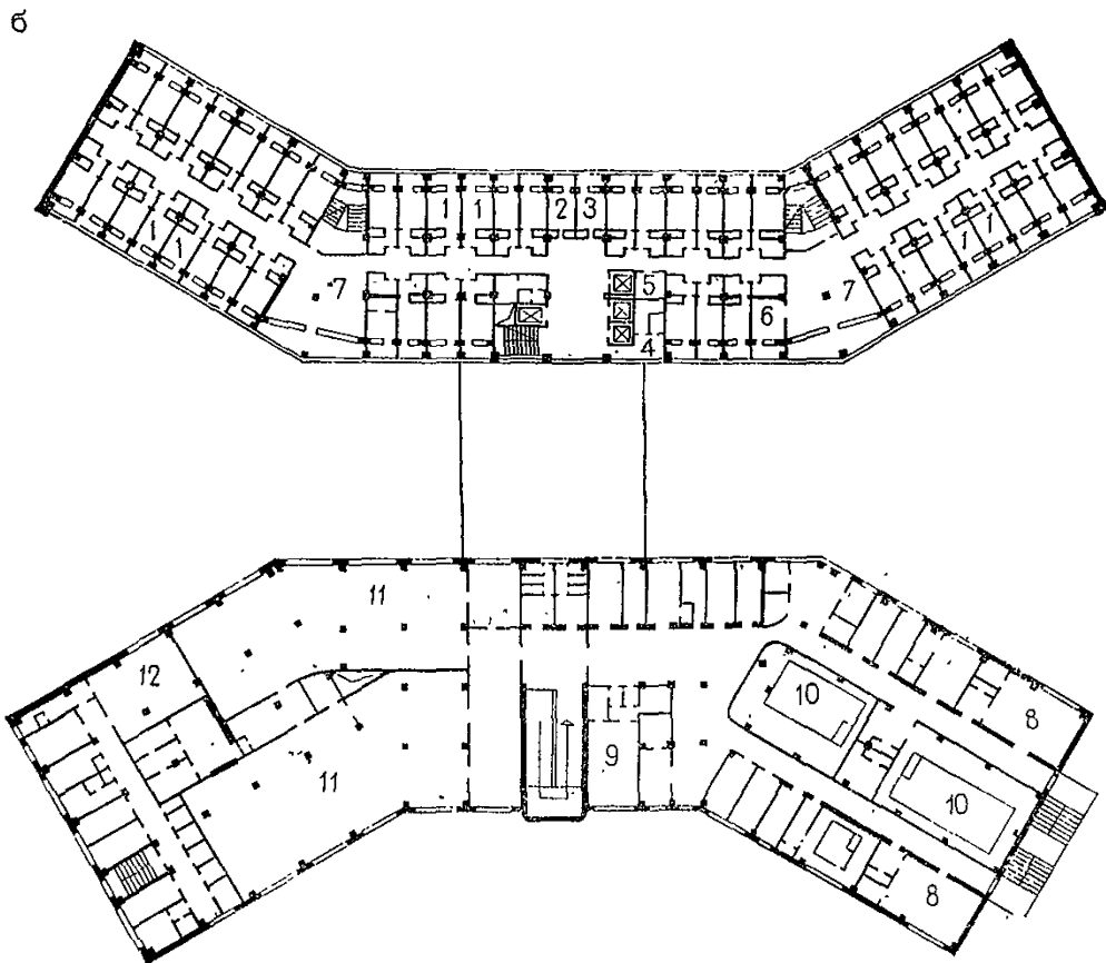
Рис. 16. Санаторий «Приморье» на 500 мест в Евпатории
