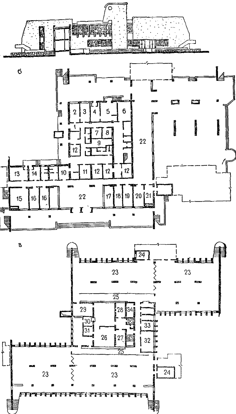
Рис. 24. Столовая на 700 посадочных мест санатория «Прибой» в Евпатории:
