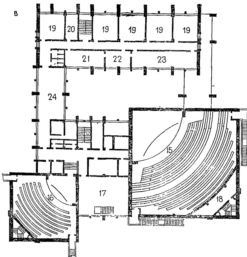
Рис. 19. Клуб межколхозного комплекса здравниц в Анапе
