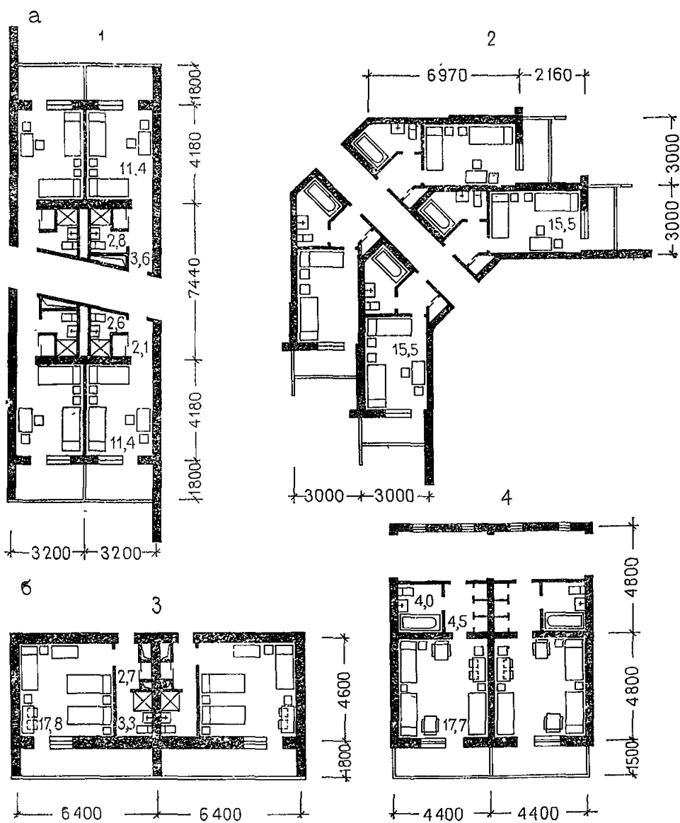
Рис. 10. Примеры планировки спальных ячеек
