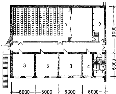
Рис. 22. Фрагмент плана 3 этажа санатория «Пролисок» в Моршине
