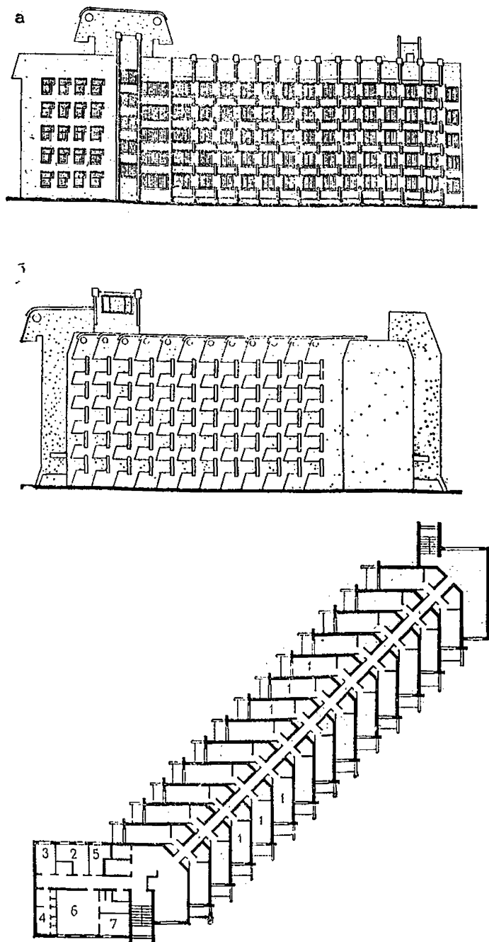
Рис. 13. Проект реконструкции и расширения санатория «Прибой» в Евпатории. Спальный корпус на 250 мест
