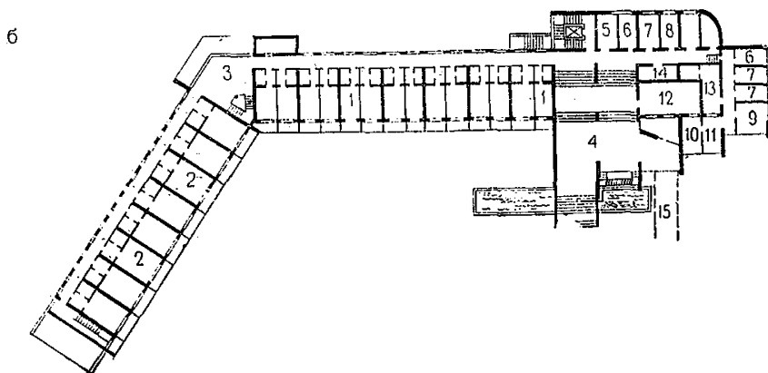
Рис. 15. Санаторий «Прогресс» в Хосте Спальный корпус на 300 мест
