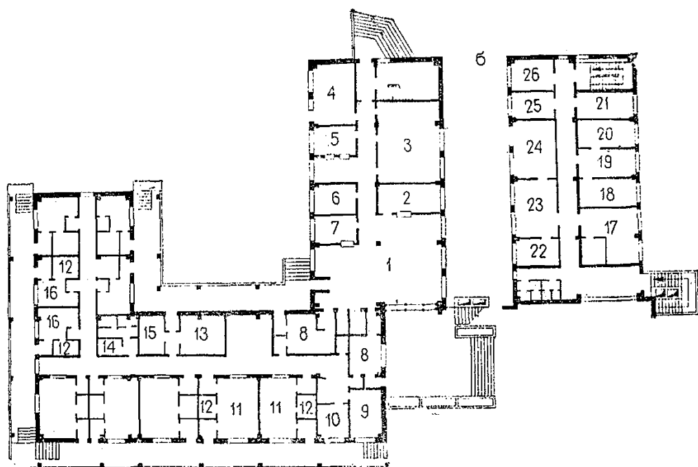
Рис. 9. Административно-приемный корпус с изолятором межколхозного комплекса здравниц для родителей с детьми в Анапе
