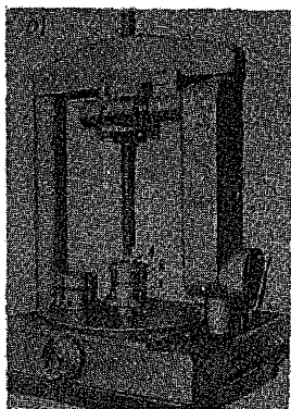
Рис. 1. Пресс ГМГ с пресс-формой конструкции Гидропроекта в разобранном (а) и собранном виде
