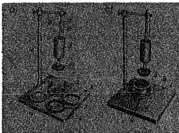
Рис. 2. Прибор стандартного уплотнения в разобранном (а) и собранном (б) виде
