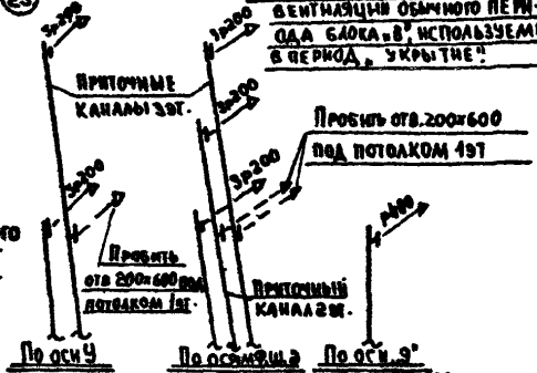
Выкопировка из схем систем приточной вентиляции блока „В“
