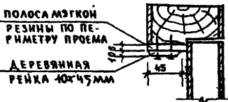
ДЕТАЛЬ УПЛОТНЕНИЯ ДВЕРНОГО ПРОЕМА
