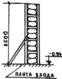
ДЕТАЛЬ УПЛОТНЕНИЯ ДВЕРНОГО ПРОЕМА
