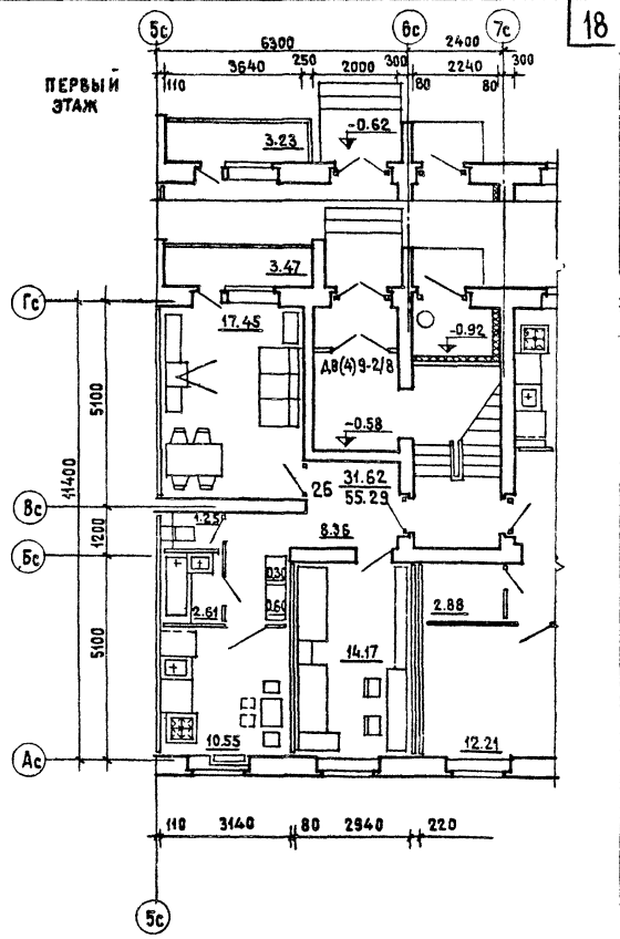
Блок-секция 86-010/А. Секция 3Б-5А. Типовой этаж. Фрагмент секции 1 этажа
