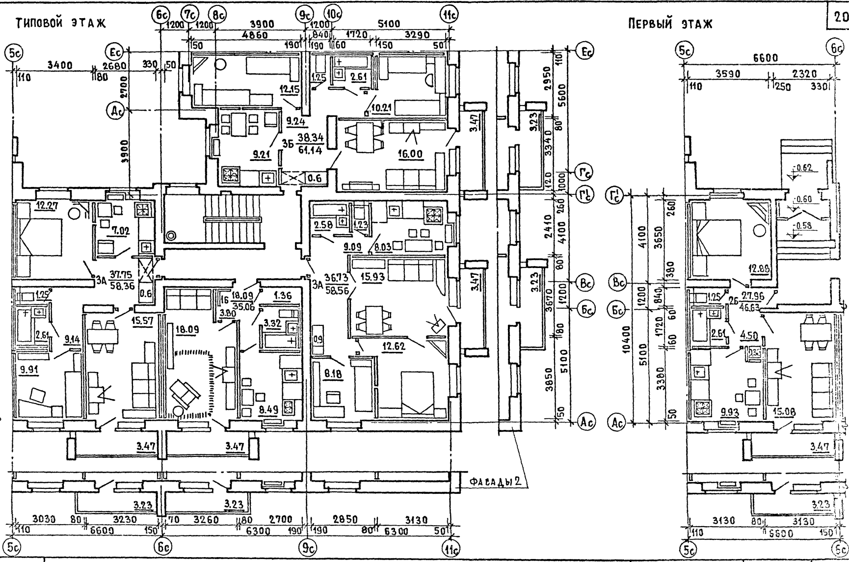
1980 Блок-секция 86-022/1. Секция 1Б-3А-3А-5Б/ПРАВАЯ/. ТИПОВОЙ ЭТАЖ. ФРАГМЕНТ СЕКЦИИ 1 ЭТАЖА.
