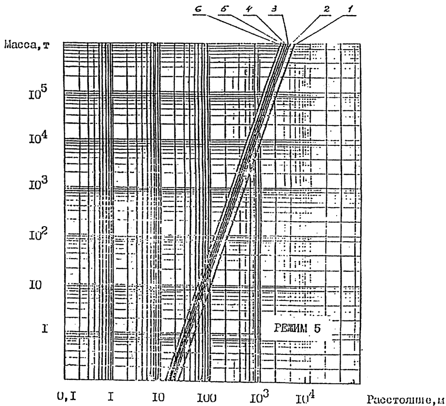
Рис. 4.12. Границы зон поражения льдом при взрывах облаков ТЛС.
