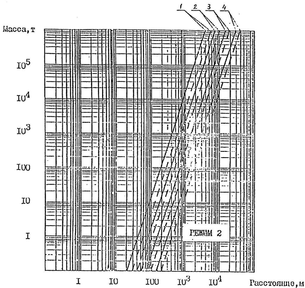
Рис. 4.3. Зависимость стеновой разрушения зданий от массы топлива и расстояния.
