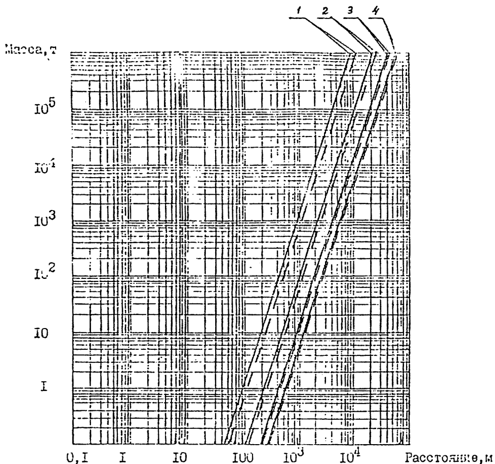
Рис. 7.1. Зависимости степеней разрушения зданий от масс и расстояния для I-го класса КВВ:
