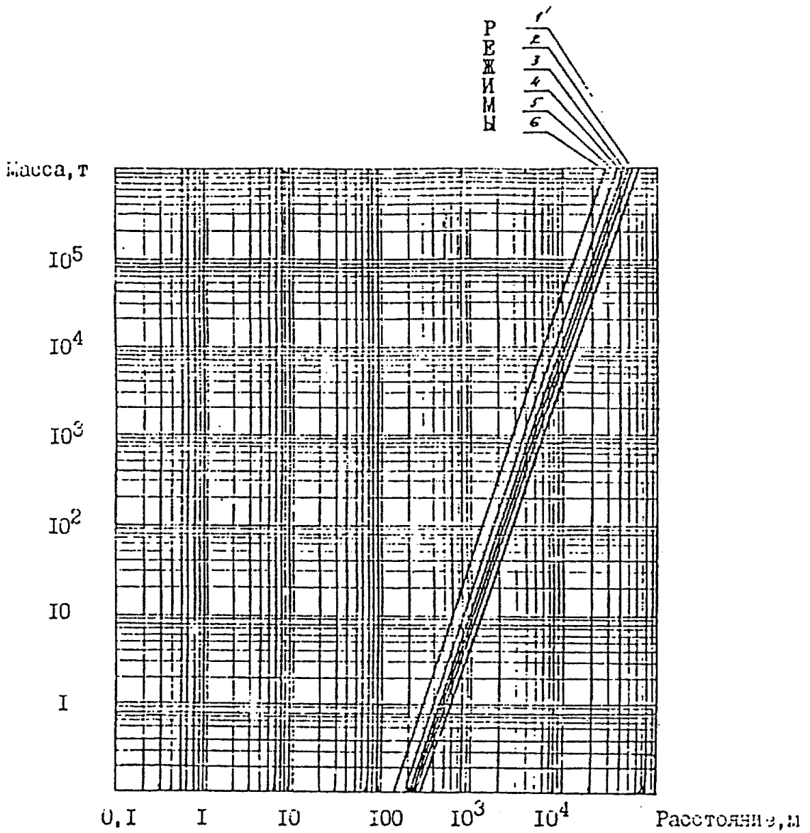
Рис. 4.14. Размеры зоны расстворения при различных режимах взрывного превращения облака ТВС
