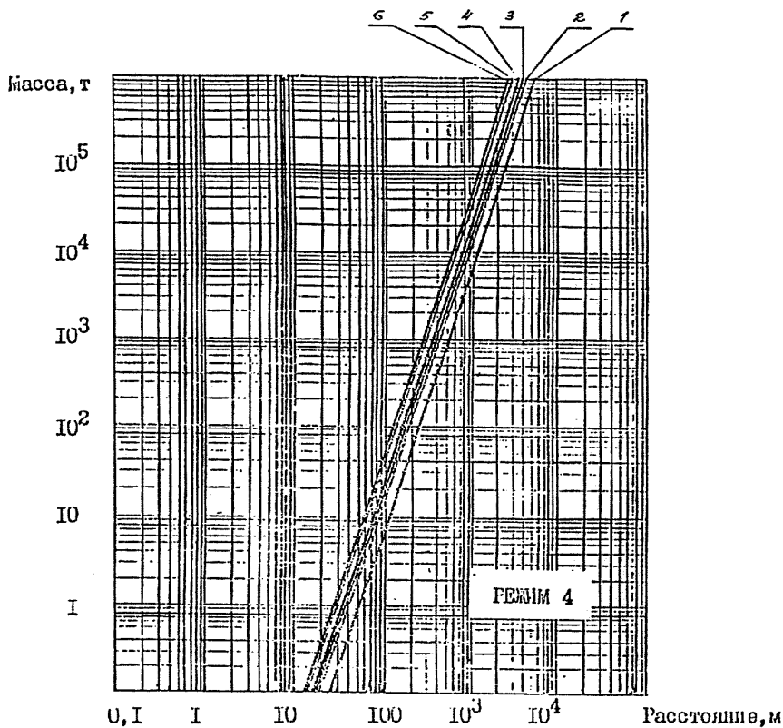
Рис. 4.11. Границы зон поражения льдов при взрывах облаков ТЦС.
