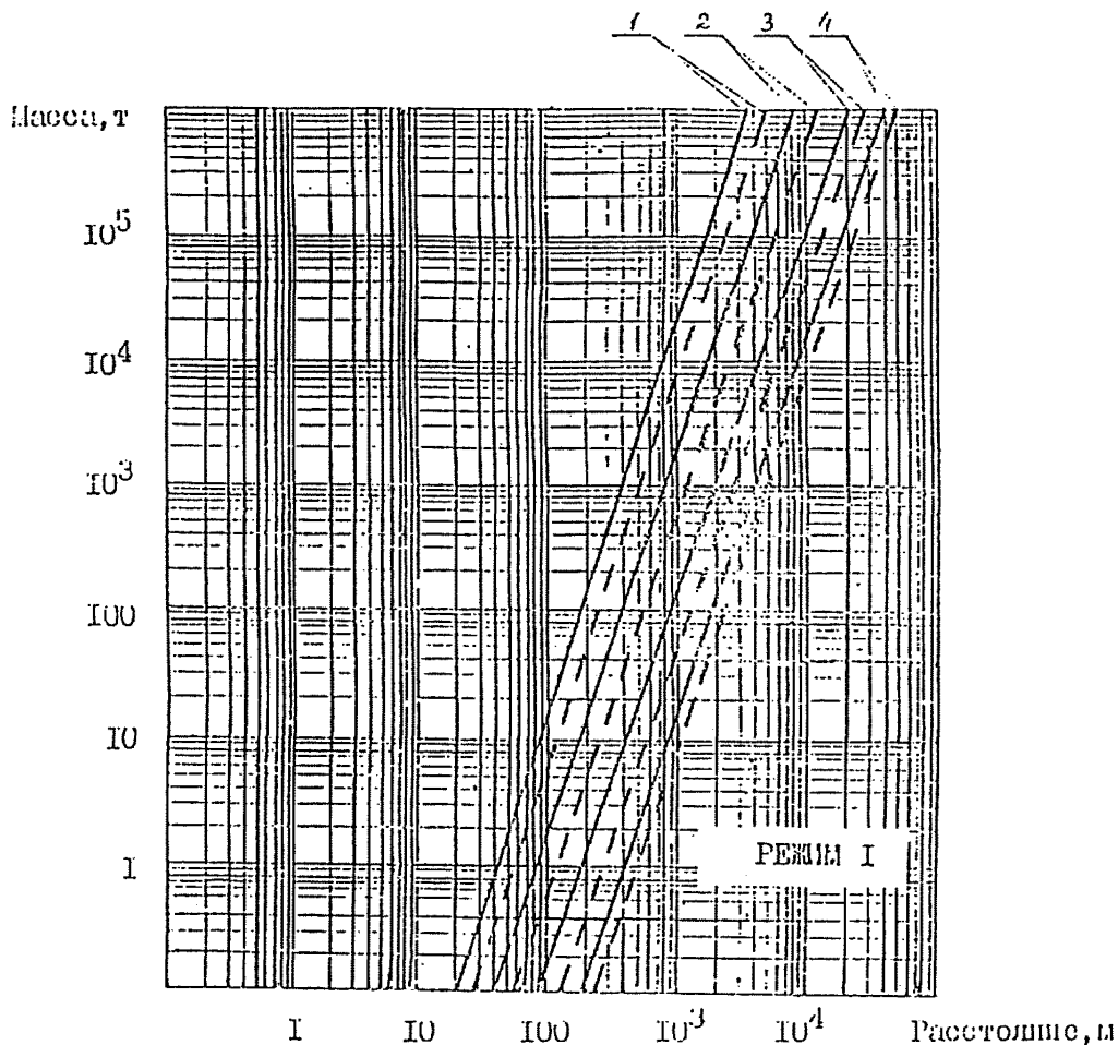
Рис. 4.2. Зависимость степени разрушения зданий от массы толщеа и расстояния.
