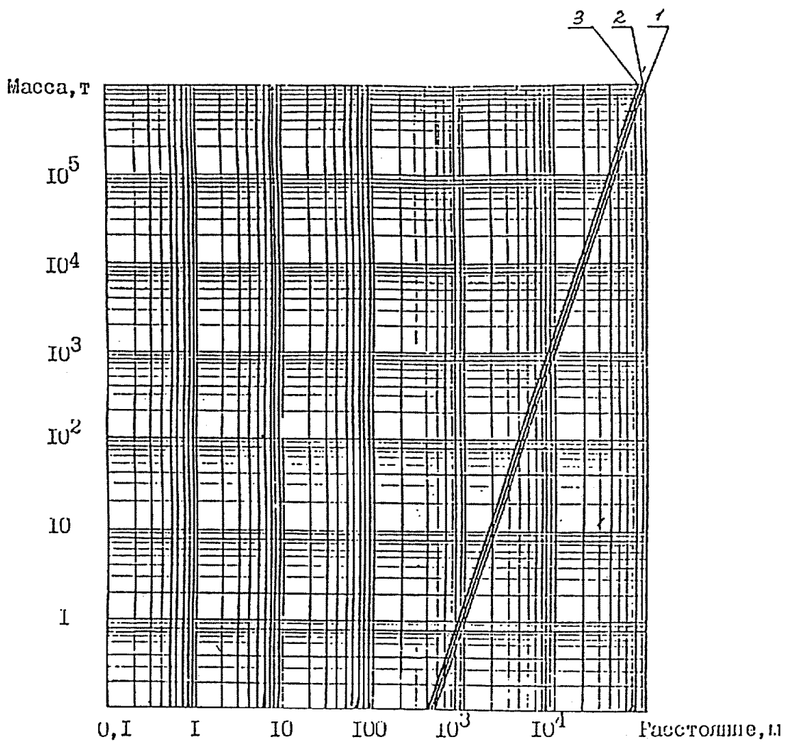
Рис. 7.4. Размеры зоны расстреливания при взрывах КВВ разных классов
