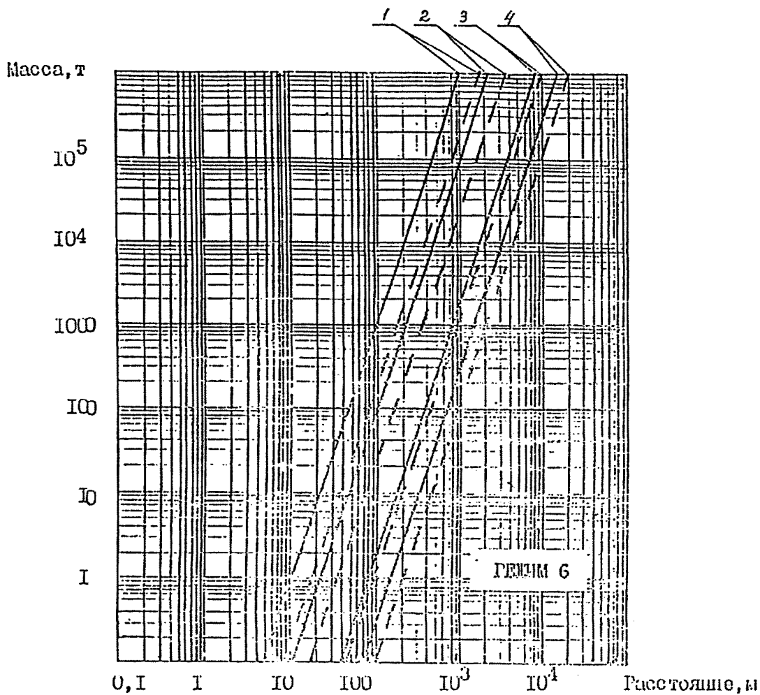
Рис. 4.7. Зависимость степеней разрушения зданий от массы бомбы и расстояния.
