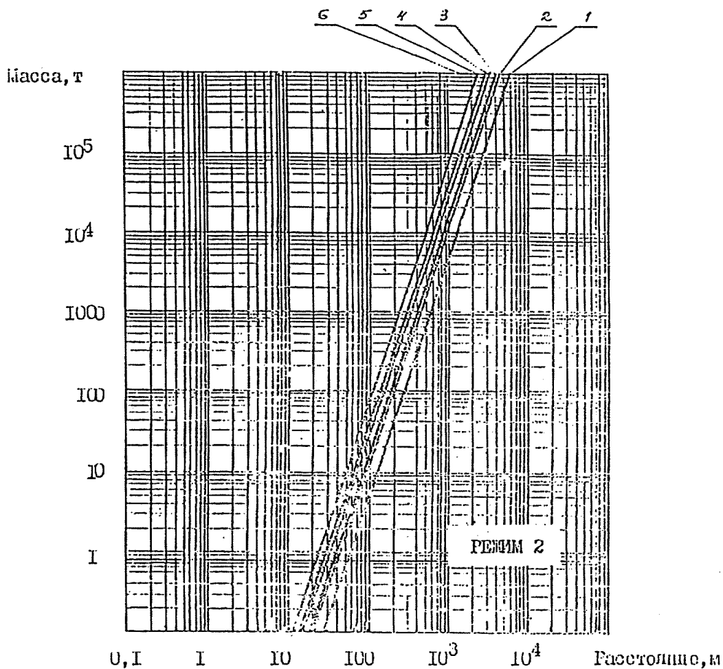
Рис. 4.9. Границы зон поражения людей при взрывах облаков ТЭС.
