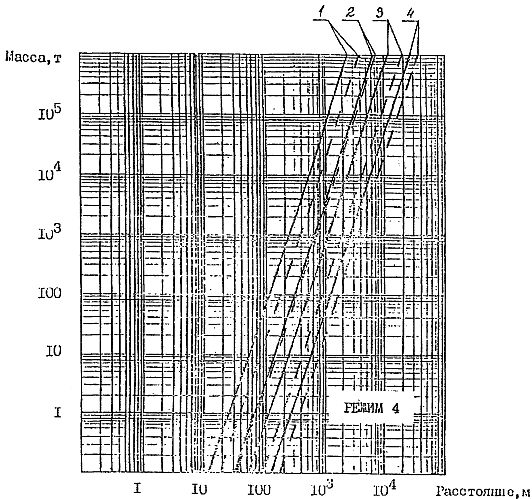
Рис. 4.5. Зависимость степеней разрушения зданий от массы толщева и расстояния.
