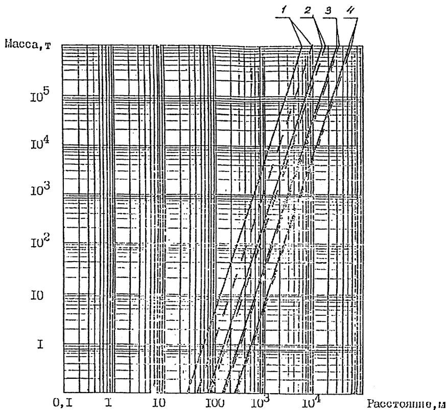
Рис. 7.3. Зависимости степеней разрушения зданий от массы и расстояния для 3-го класса (ВВ):
