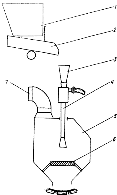
Рис.1. Схема пневмоударной установки:
