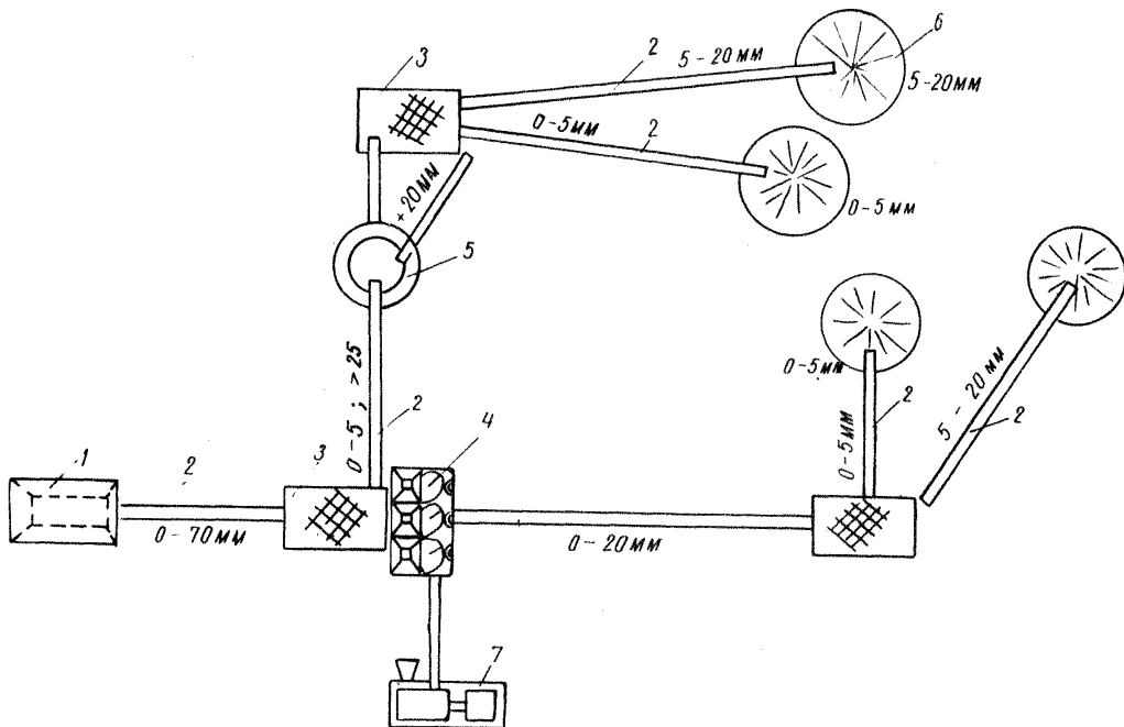
Рис.2. Схема переработки гравия на пневмоударной и конусной дробилках : 1-бункер-питатель; 2-ленточный конвейер; 3-грохот; 4-пневмоударная установка; 5-конусная дробилка ; 6-склад; 7-воздуходувка
