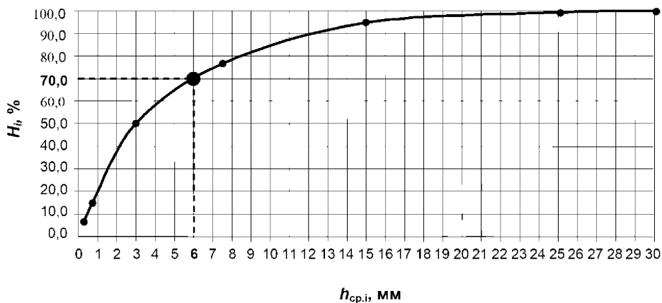
Рисунок И.1 Зависимость принимаемого на очистку суммарного за год слоя жидких осадков (%) от величины максимального суточного слоя дождя (мм), принимаемого на очистку в полном объеме, для г. Санкт-Петербург (по метеостанции Ленинград, ИЦП)
