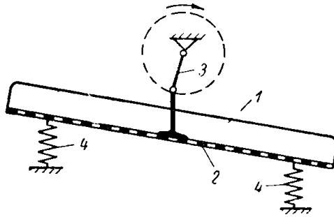
Рис. 4. Схема одношального гирационного грохота 1 — короб; 2 — сито; 3 — кривошип; 4 — упругие опоры
