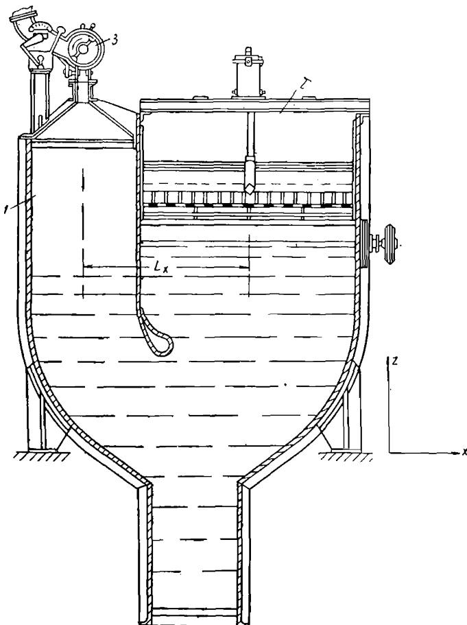
Рис. 8. Схема устройства беспоршневой отсадочной ма- шины 1 — воздушное отделение; 2 — ситовое отделение; 3 — золотнико- вое устройство
