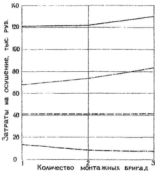
Рис.2. Затраты на осушение в зависимости от варианта резервирования. Приведенные капитальные затраты: --- на сооружение основных скважин; ---- на сооружение резервных скважин; ..... эксплуатационные затраты; — суммарные приведенные затраты.
