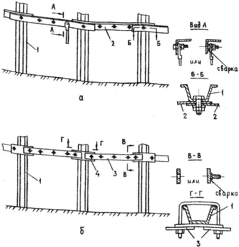
Рис.5. Пример устройства местного заземлителя в камерах, местах уширений штрехов и других стационарных условиях а)- с использованием специально изготовленных стяжек из уголка при применении крепи, имеющей отверстия для закрепления стяжек; б)- с использованием специальных стяжек из полосы: I - стойна крепи; 2 - специальный стяжной элемент из уголка с отверстиями или шпильными для присоединения заземляющих проводников, 3 - из полосы; 4 - планна
