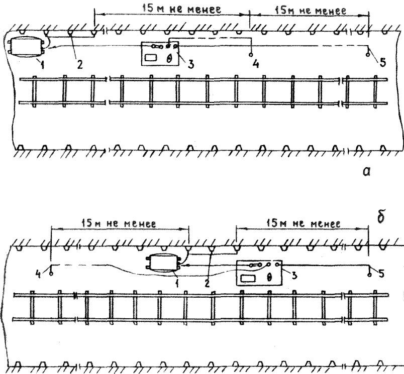
Рис.7. Пример расположения измерительных электродов при контроле сопротивления заземления а)- при расположении электродов по одну сторону от заземленного объекта; б)- по разные стороны:
