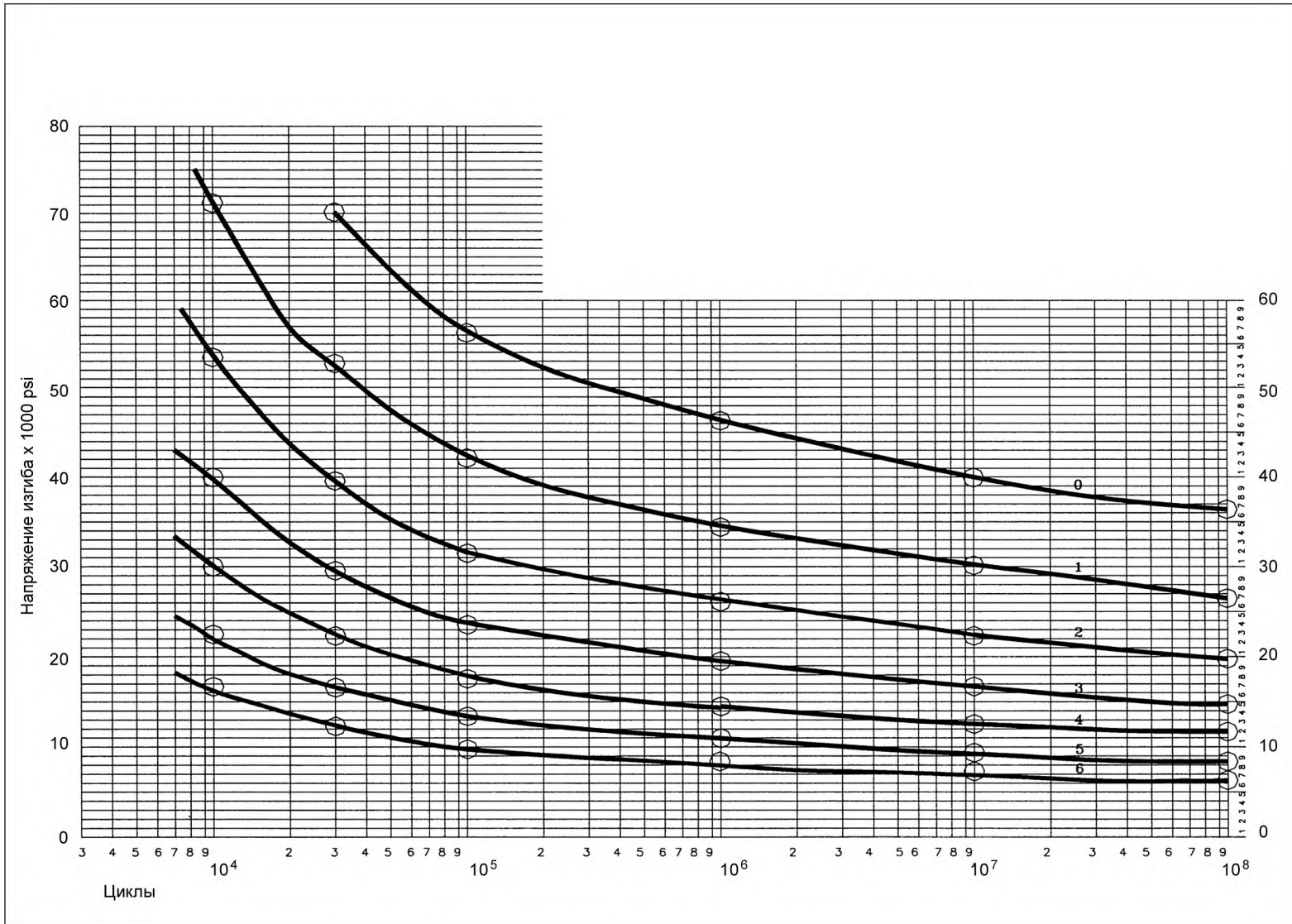
Рисунок 1 — S/N кривая испытания на усталостное разрушение при изгибе
