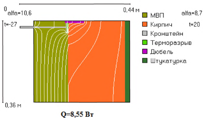
Рисунок 12.1 – Температурное поле узла конструкции, содержащего кронштейн
