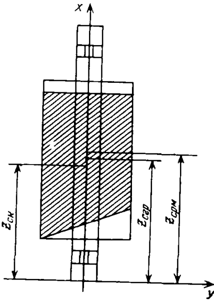
Рис.Д.3.9 Расчетная схема к определению центральных моментов инерции подъемного сосуда
