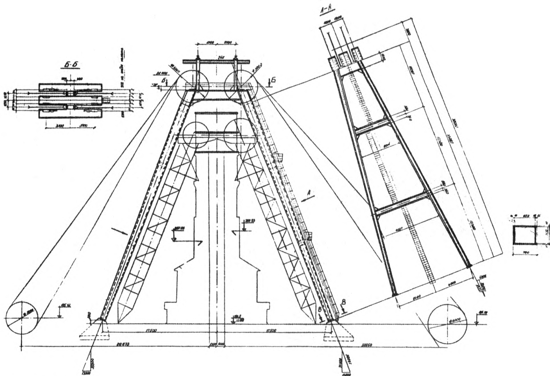
Рис. II.7. I. Схема подъема
