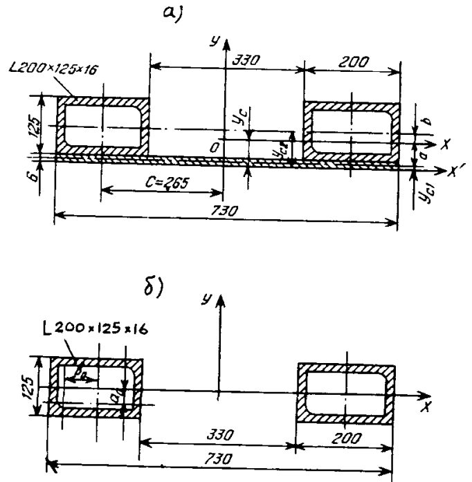
Рис.Д.3.10 Поперечные сечения рамы скана выше (а) и ниже (б) кузова
