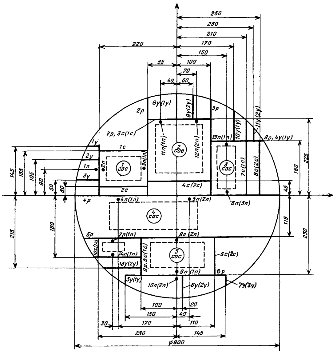
Рис. П.2.13. Условная формализованная технологическая схема армировки отвода
