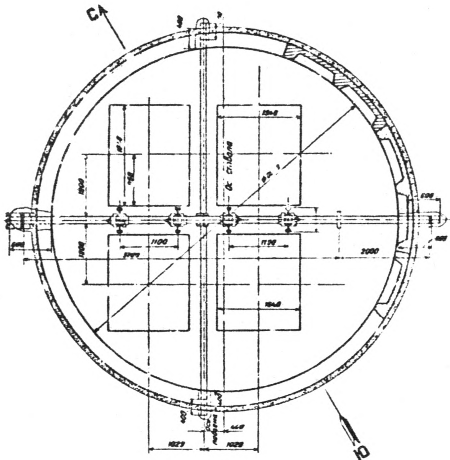
РИС. П. 7. 4. СЕЧЕНИЕ СТВОЛА ПРОЕКТИРЪЕМЪЕ
