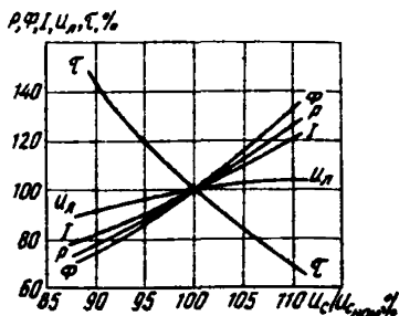
Рис. 3. Зависимость параметров лампы ДРЛ от напряжения питания R — мощность лампы; \Phi — световой поток лампы; I — ток лампы; U_l — напряжение на лампе; \tau — продолжительность горения
