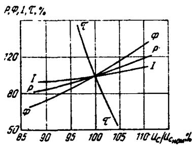
Рис. 2. Зависимость параметров лампы накаливания от напряжения питания R — мощность лампы; \Phi — световой поток лампы; I — ток лампы; \tau — продолжительность горения
