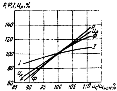
Рис. 4. Зависимость параметров лампы ДНаТ от напряжения питания P — мощность лампы; \Phi — световой поток лампы; I — ток лампы; U_L — напряжение на лампе
