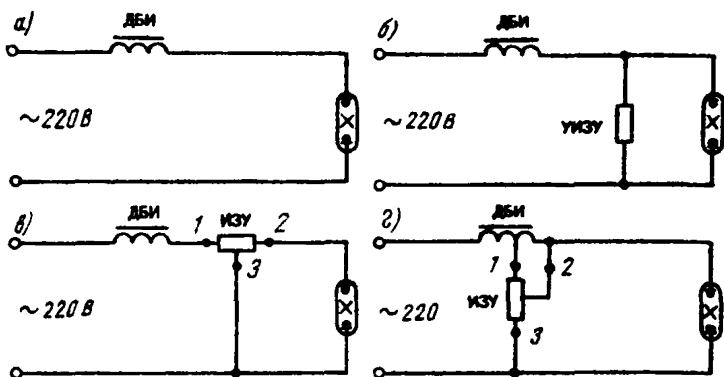
Рис. 1. Схемы включения газоразрядных ламп высокого давления и ламп ДРЛ; б, в, г — лампы ДНАТ (ДРИ) с импульсными зажигающими устройствами; 1, 2, 3 — нумерация вводимых клемм ИЗУ
