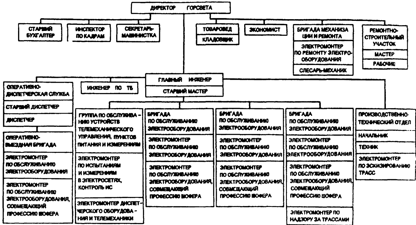
Рис. 2. Примерная организационная структура предприятия горсвета для города с населением 250 тыс. жителей, освещаемого 7500 светильниками при объеме работы в 2500 условных единиц
