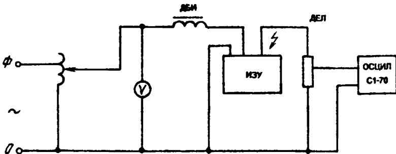
Рис. 1. Схема проверки электрических параметров импульсных зажигающих устройств T — автотрансформатор лабораторный типа ЛАТР-1М; V — вольтметр класса точности 0,5; ДБИ — дроссель балластный; ИЗУ — импульсное зажигающее устройство; Осцил — осциллограф С1-70 или ему подобный; Дел — делитель напряжения
