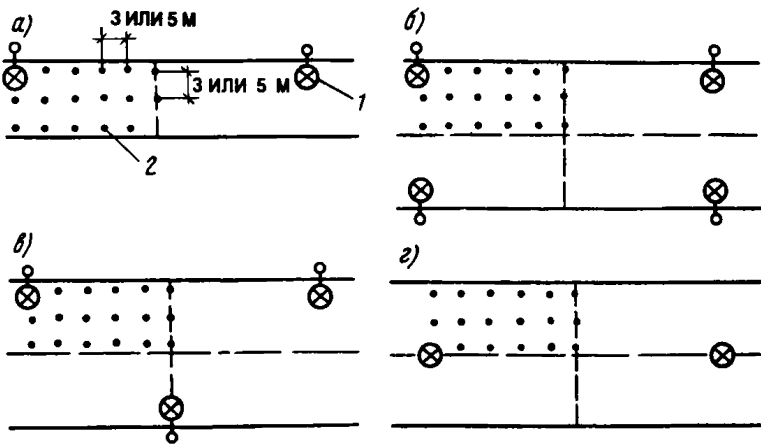
Рис. 1. Размещение точек измерения освещенности для определения средней освещенности или средней яркости косвенным методом при различном расположении светильников
