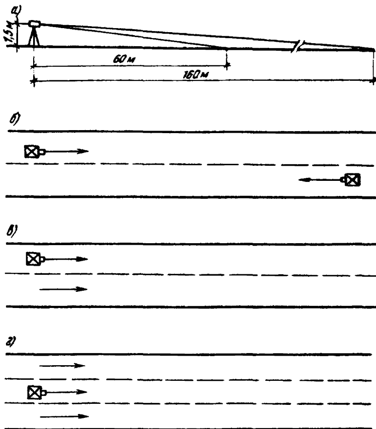
Рис. 2. Положение яркомера при измерении яркости покрытий дороги в зависимости от числа полос и направлений движения а — установка яркомера; б — дорога с двумя полосами, движение двустороннее; в — дорога с двумя полосами, движение одностороннее; г — дорога с тремя полосами, движение одностороннее
