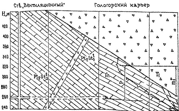
Разрез по I-I
