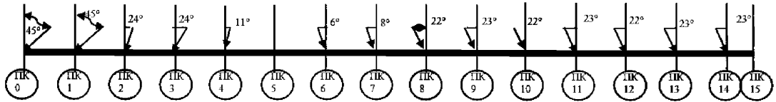
Рис. 4.3.1-2 Направление скоростей течения/волн относительно участков трассы морского трубопровода
