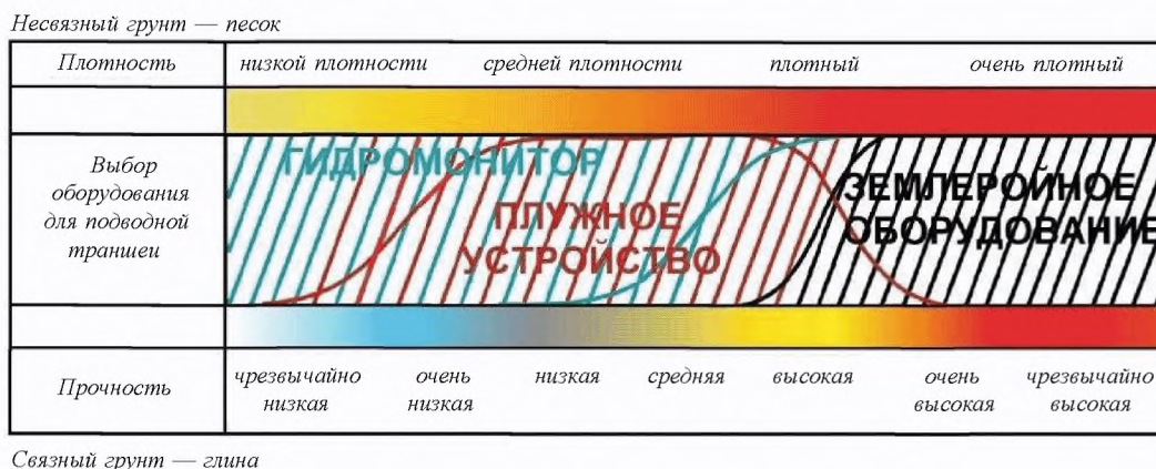
Рис. 10.2-3 Выбор технологии подготовки подводной траншеи [1]
