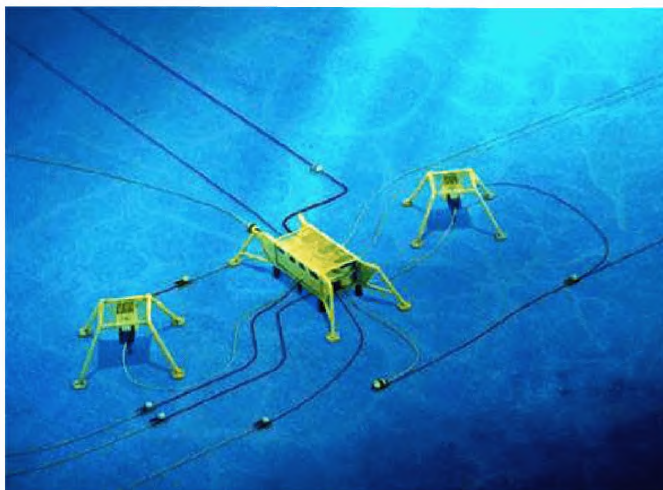
Рис. 3.1 Подводный добывающий комплекс (СПДК) и подводные трубопроводы (МПП): манифольд, добычные скважины с подводным расположением устья с защитными конструкциями и подводные трубопроводы [2]
