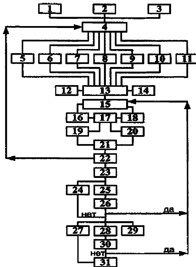
Рис. 2.4 Общие принципы проектирования подводного трубопровода [13]:
