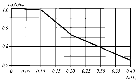
Рис. 7 Зависимость c_v(\Delta)/c_v от относительного заглубления трубопровода \Delta/D_a
