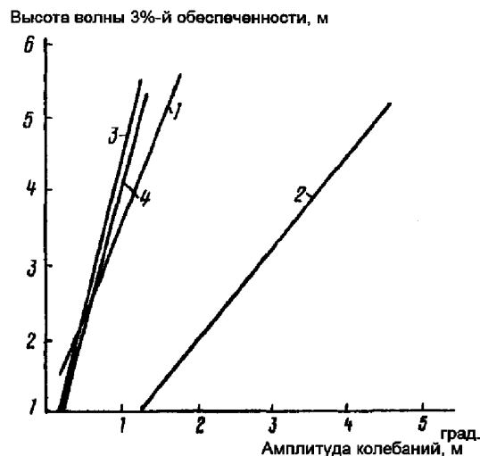
Рис. 7.3-1 Амплитуды качки на нерегулярном волнении 3%-й обеспеченности ТУС SULEYMAN VEZIROV [2]: 1, 2 — килевая ( \psi ) и бортовая ( \theta ) качка; 3, 4 — горизонтальная ( a_g ) и вертикальная ( a_v ) качка
