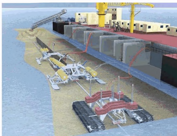
Рис. 7.6-3 Комплексное устройство для заглабления и обратной засыпки подводного трубопровода компании Saipem S.p.A.
