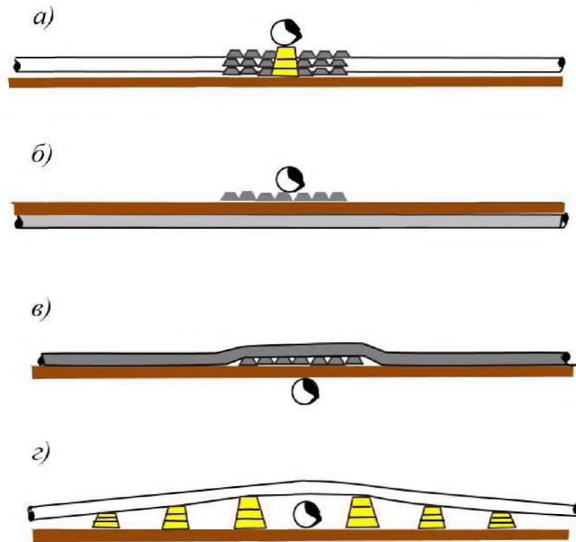
Рис. 11.2-1 Примеры пересечений подводных трубопроводов [1]:
