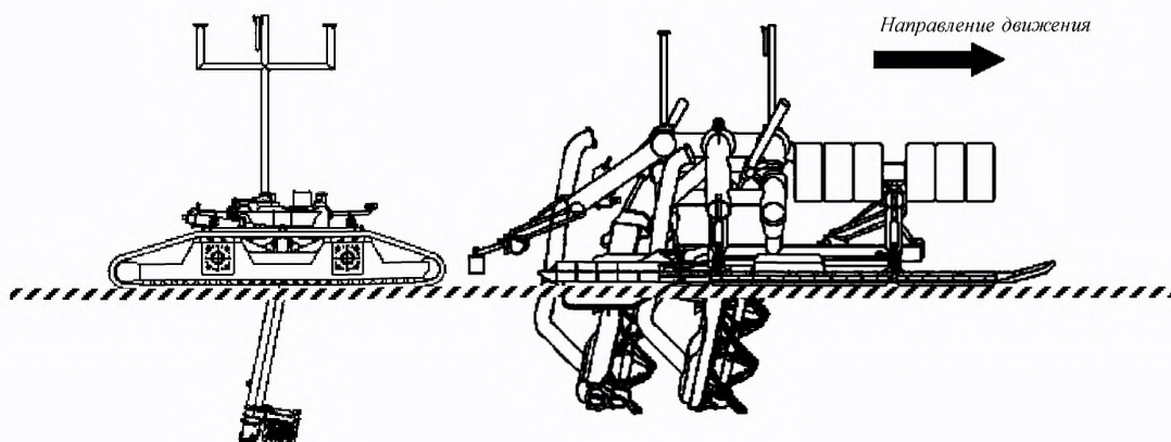
Рис. 7.6-2 Устройство заглабления подводного трубопровода компании Saipem S.p.A.
