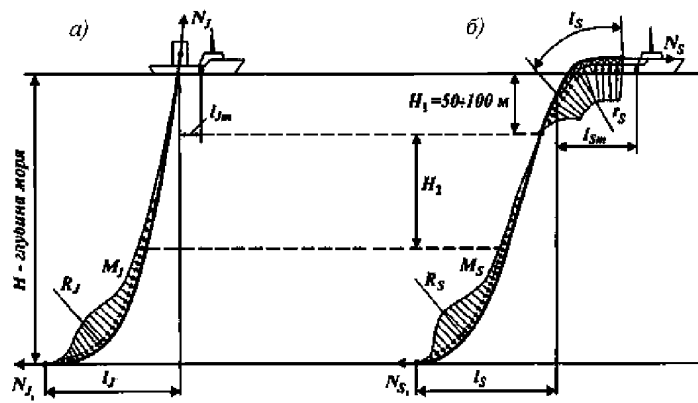
Рис. 7.1-3 Эпюры изгибающих моментов при укладке различными способами [1]: a — J -метод укладки; б — S -метод укладки
