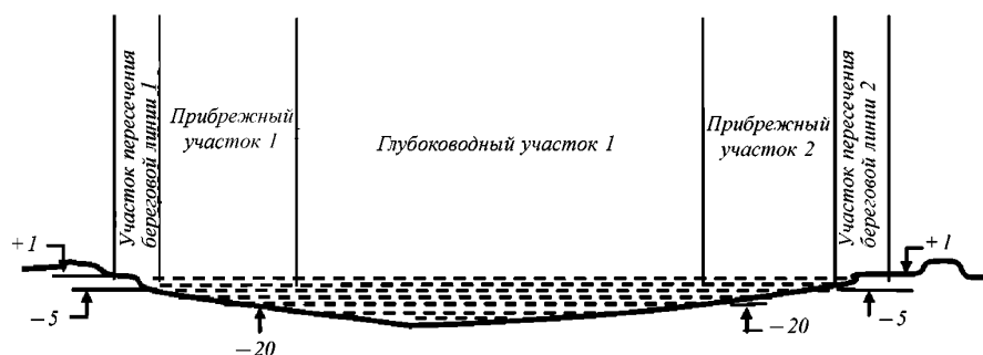
Рис. 10.1-1 Участки трассы морского трубопровода [3]
