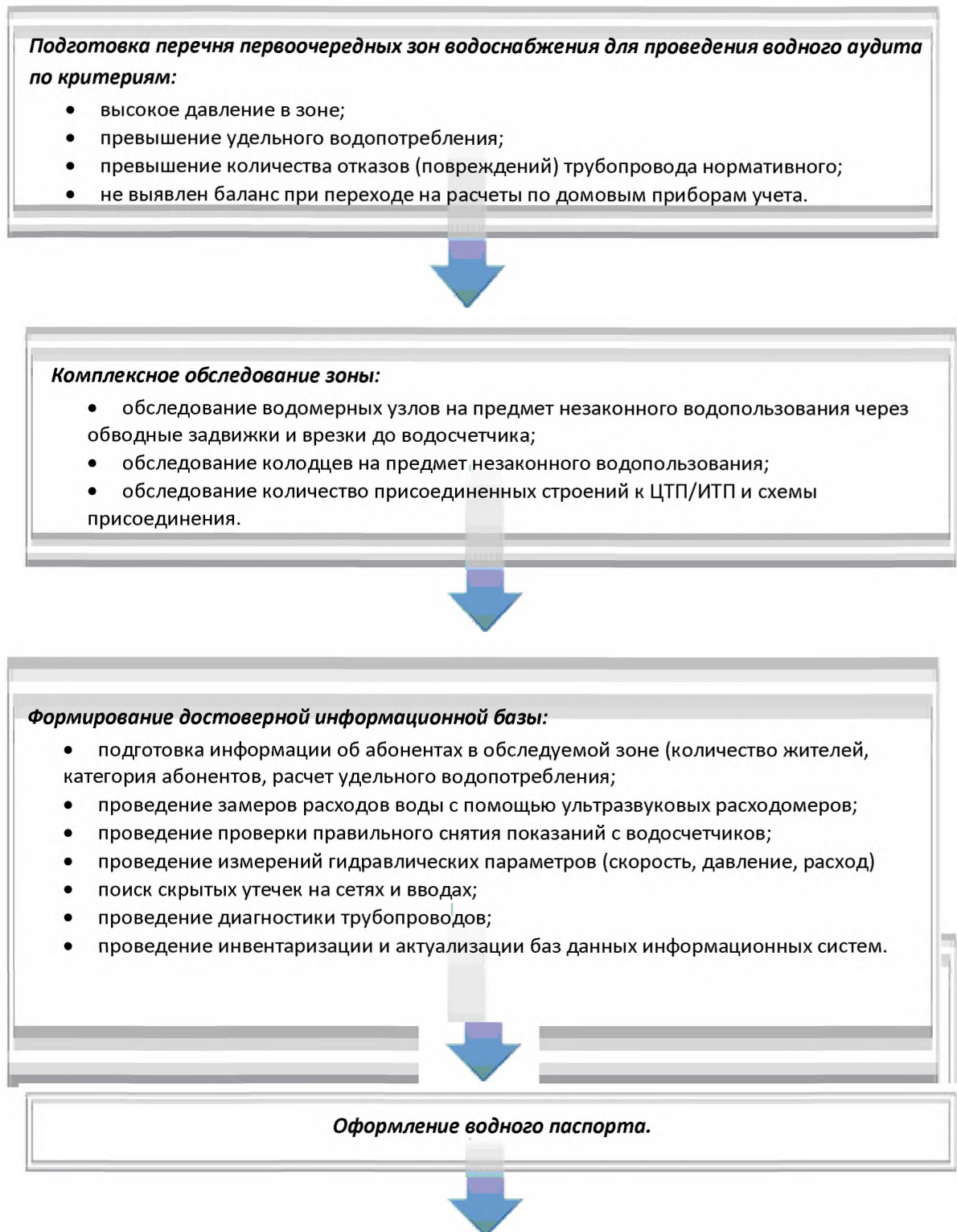
Рисунок 7.3 – Пошаговая методика проведения водного аудита
