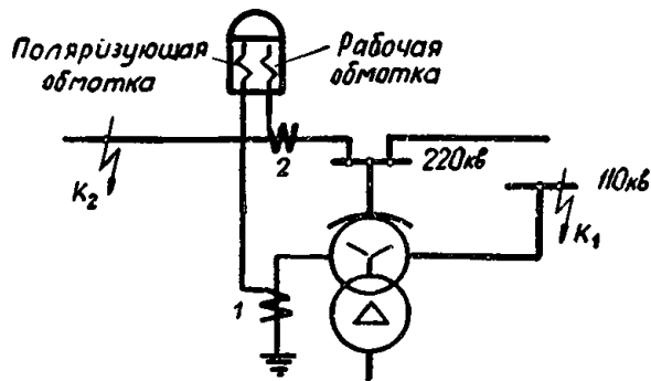
а) Схема включения реле
