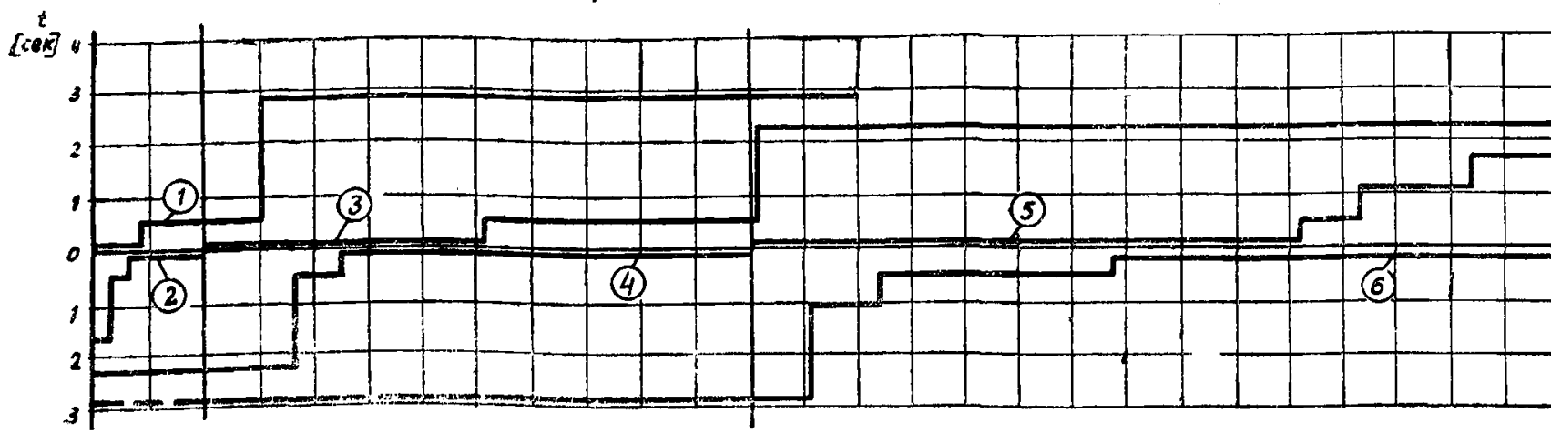
Рис. 22. Защищаемые зоны первых и вторых ступеней защит 1—6 и третьих ступеней защит 5 и 6 в сети рис. 19.
