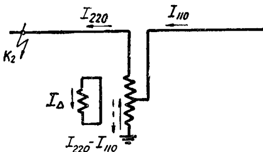
в) Замыкание в точке K_2 (схемы "а")
