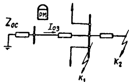
а) Расчетная схема замещения нулевой последовательности.
