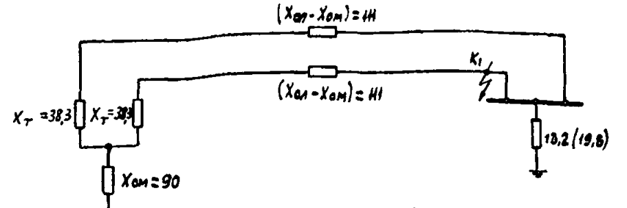
в-1) Схема замещения нулевой последовательности при к.з. на землю в точке K_1
