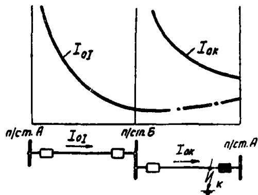
в) Пример изменения токов в поврежденной и неповрежденной линиях.
