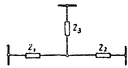
б) Исходная схема и схема замещения двух параллельных линий, одна из которых имеет заход шлейфом на подстанцию, а другая заземлена с обоих концов.
