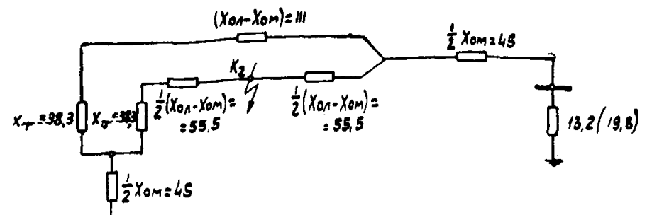
в-2) Схема замещения нулевой последовательности при к.з. на землю в точке K_2
