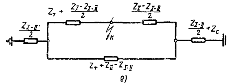
Рис. П-13. Схемы замещения нулевой последовательности двух параллельных блоков трансформатор—линия. U_A, U_B, U_B —напряжения нулевой последовательности на шинах станции и н/ст. В.
