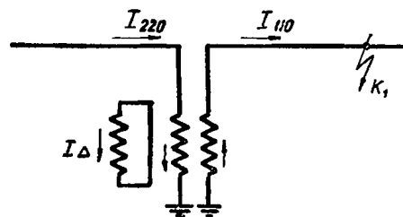
б) Замыкание в точке K_1 (схемы «а»)
