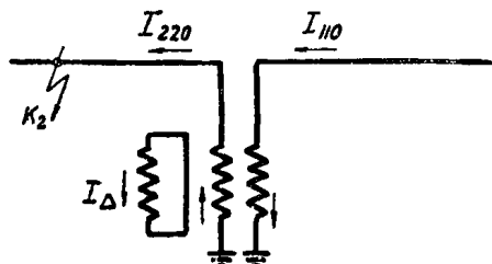
в) Замыкание в точке K_2 (схемы «а»)
