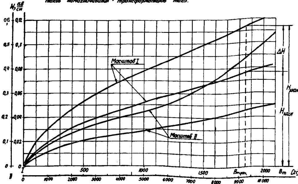
в). Предельные кривые намагничивания ленточных сердечников из трансформаторной стали марки (Э310)ХВП
