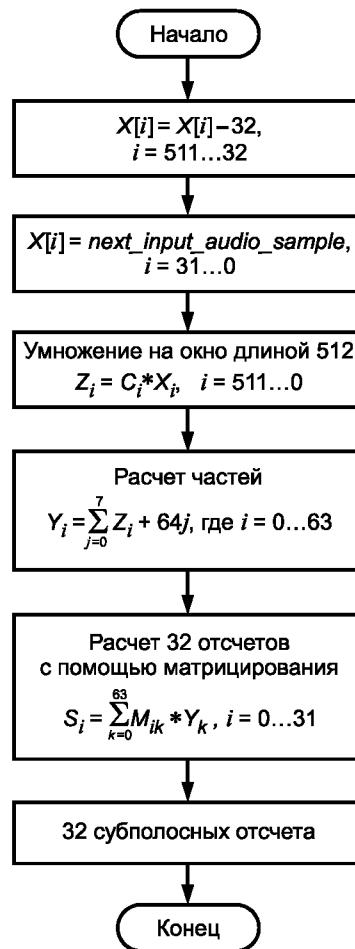
Рисунок В.4 — Блок-схема алгоритма субполосной фильтрации
