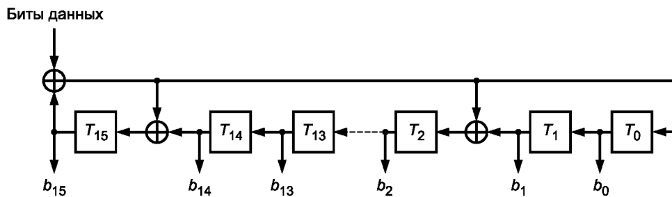
Рисунок А.9 — Схема проверки CRC
