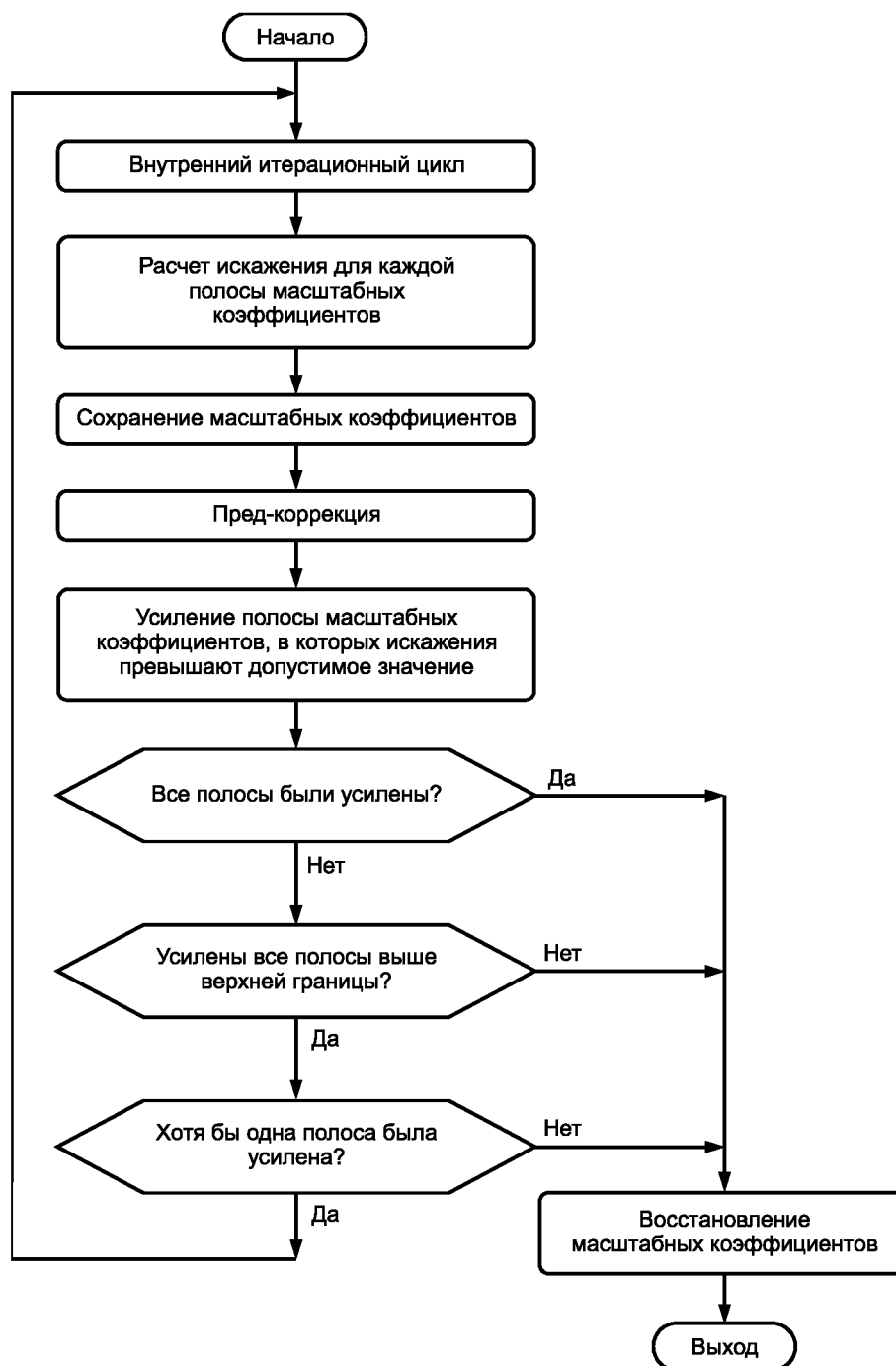
Рисунок В.96 – Внешний цикл итерации. Уровень III
