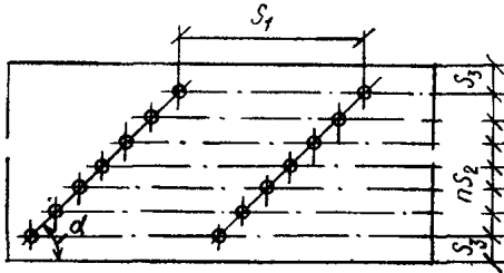
Рис. 12. Схема расстановки гвоздей косыми рядами
