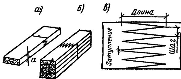
Рис. 6. Схемы зубчатых соединений
