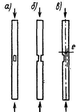
Рис. 2. Ослабления сжатых элементов
