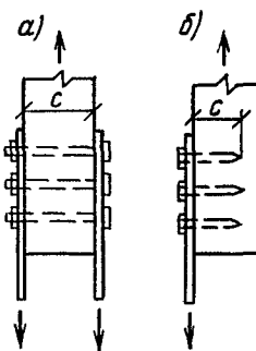
Рис. 9. Нагельные соединения со стальными накладками
