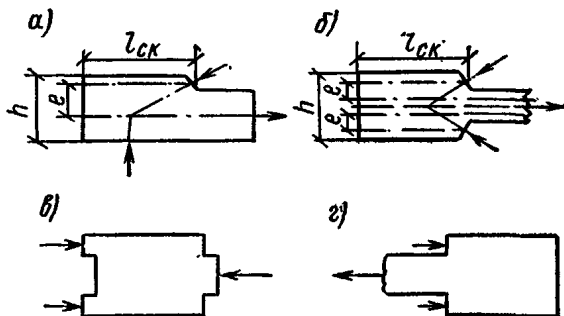
Рис. 5. Схемы врезок в элементах соединений (а и б); схемы одностороннего (с) и промежуточного (г) скалывания для случая симметричных врезок
