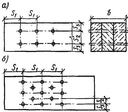
Рис. 10. Схема расстановки нагелей а — прямой; б — в шахматном порядке
