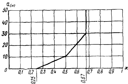
Рис. 2. График для определения значения коэффициента спада ветровой нагрузки x при зональном действии ветра
