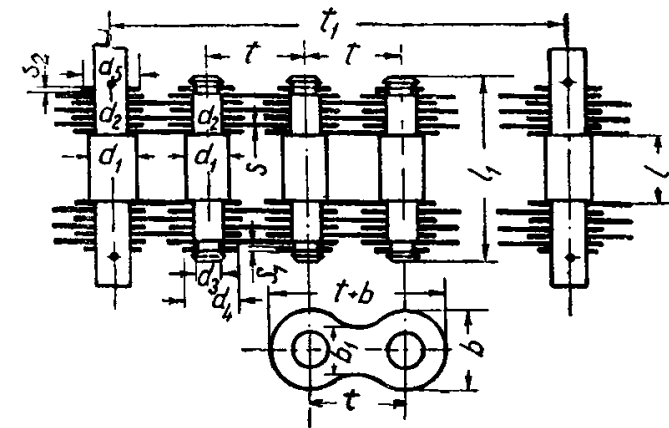
2. Цепь с расклевкой на шайбе
