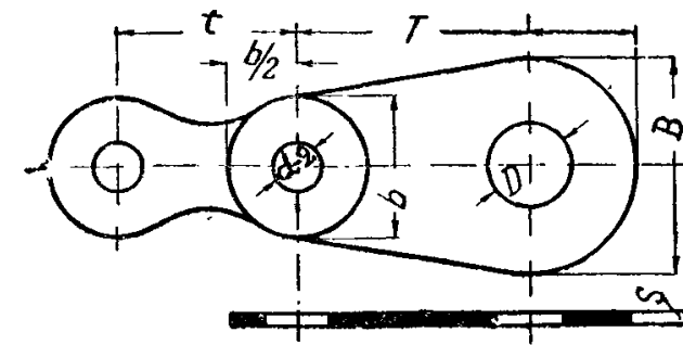
4. Концевые пластины
