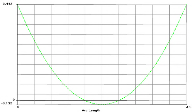
Рисунок 45–Вертикальные перемещения плиты покрытия в поперечном шве от собственного веса и воздействия температур
