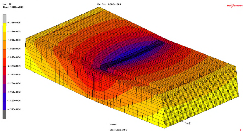
Рисунок 18– Вертикальные перемещения плит покрытия и основания от собственного веса и транспортной нагрузки в м (для наглядности перемещения увеличены в 1500 раз)
