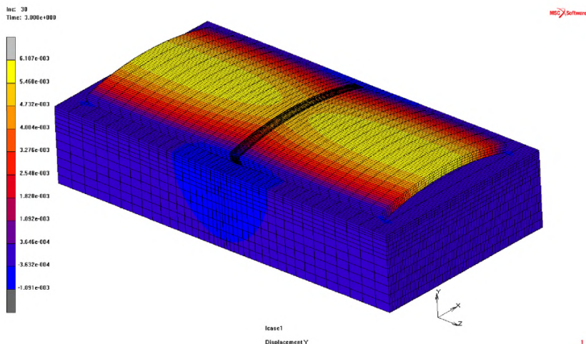
Рисунок 34–Вертикальные перемещения плит покрытия при нагреве в летний период времени (перемещения увеличены в 50 раз)
