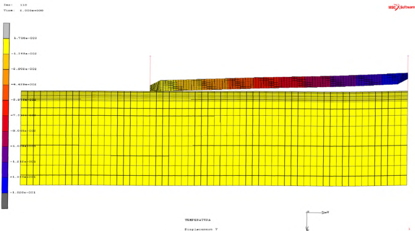
Рисунок 72 - Вертикальные перемещения плиты в конце итерационного процесса при глубине разрушения поперечных швов 10 см
