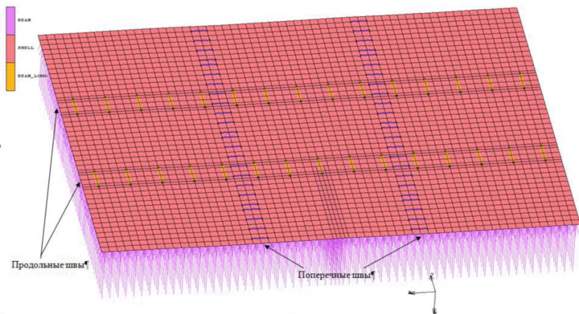
Рисунок 124—Конечно-элементная модель 3-х полосного жёсткого автомобильно-дорожного покрытия.
