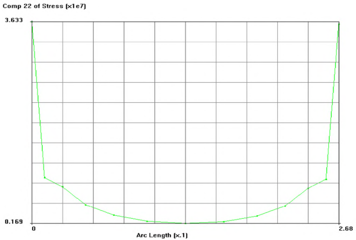
Рисунок 55–Распределение нормальных напряжений в бетоне плиты на горизонтальных площадках в окрестности стального штыря
