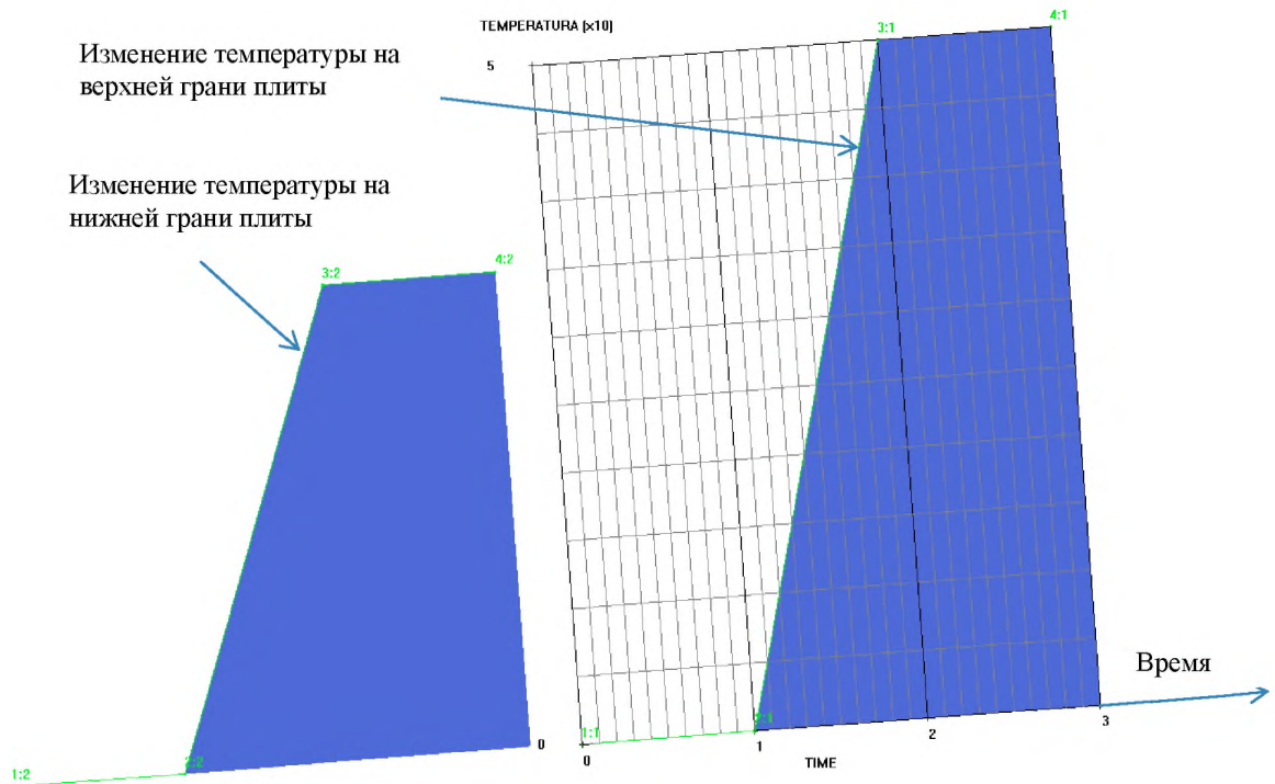
Рисунок 88 - Пространственные диаграммы изменения температуры по толщине плиты и во времени
