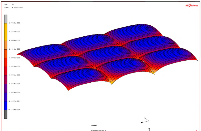
Рисунок 144– Распределение вертикальных перемещений трёхполосного жёсткого дорожного покрытия, возникающих от транспортной нагрузки на краях плиты и температурного воздействия
