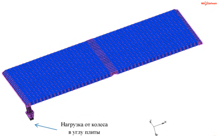
Рисунок 102 - Загружение плиты, примыкающей к обочине, давлением от колеса в углу плиты
