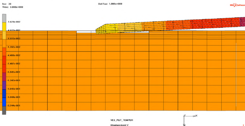
Рисунок 119 - Фрагмент распределения вертикальных перемещений плит покрытия в момент потери устойчивости с транспортной нагрузкой
