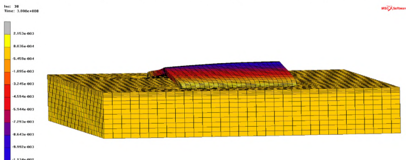
Рисунок 99 - Вертикальные перемещения покрытия от температурного воздействия при запрете горизонтальных перемещений в продольном шве (для наглядности перемещения увеличены в 60 раз)
