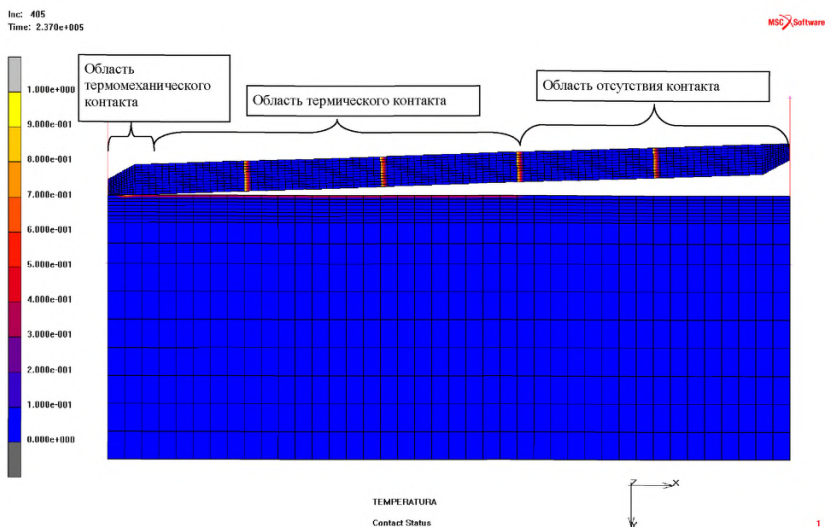
Рисунок 78– Реализация трёх видов контакта между бетонной плитой покрытия и основанием
