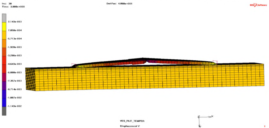
Рисунок 122 - Вертикальные перемещения покрытия от температурного воздействия при запрете горизонтальных перемещений в продольном шве (для наглядности перемещения увеличены в 40 раз)
