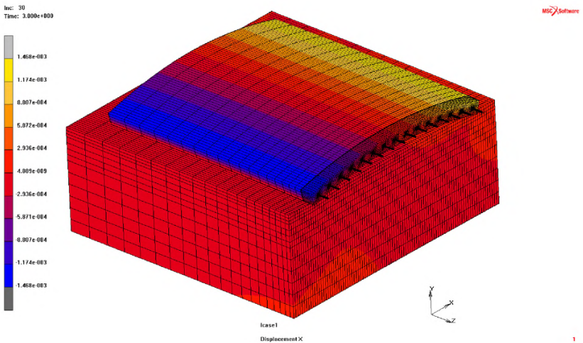
Рисунок 36–Перемещения одной из плит покрытия при нагреве в летний период времени в поперечном направлении (перемещения увеличены в 50 раз)
