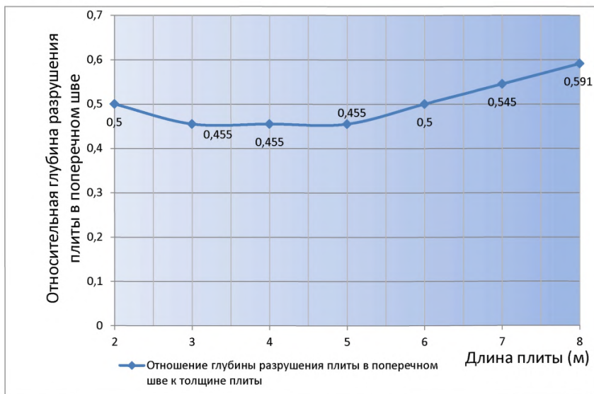
Рисунок 75– Зависимость между длиной плиты и минимальным её ослаблением в поперечном шве, при котором происходит потеря устойчивости дорожным покрытием
