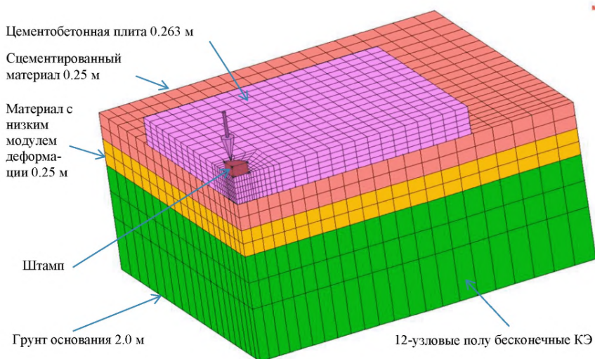
Рисунок 7 – Конечнo-элементная модель дорожного покрытия, созданная в КЭ комплексе «MARC-MENTAT»
