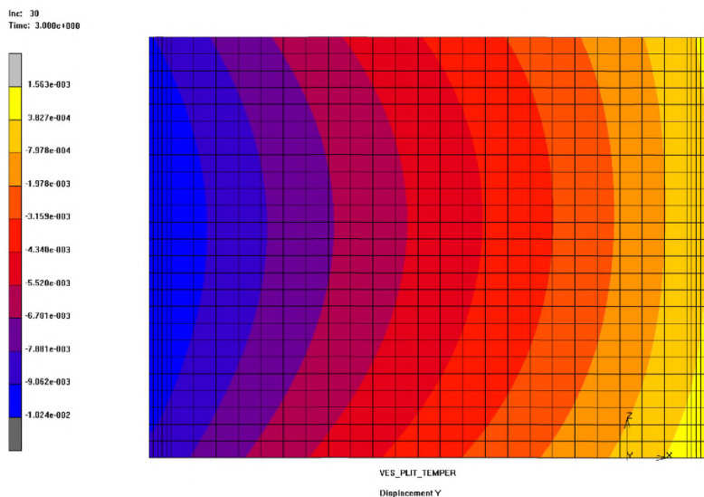
Рисунок 97 - Распределение вертикальных перемещения правой плиты
