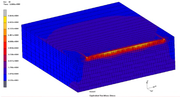
Рисунок 23—Распределение эквивалентных напряжений в основании плиты покрытия
