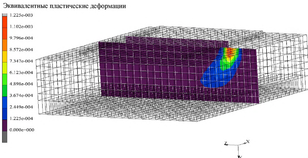
Рисунок 4 – Распределение эквивалентных пластических деформаций в упруго-пластическом основании в вертикальном сечении между узлами 2585 и 2607 (рисунок 1) при нагрузке, приложенной в середине длинного края плиты
