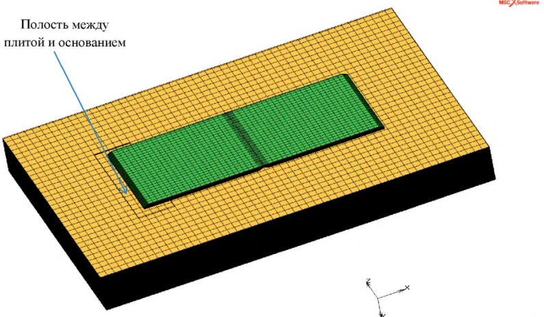
Рисунок 114 - Конечно-элементная модель жёсткого цементобетонного дорожного покрытия с полостью между плитой и основанием
