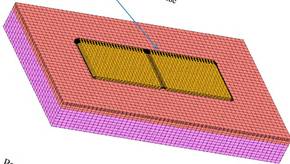
Рисунок 90 - Расчётная схема покрытия с незакреплёнными краями плит в продольных швах
