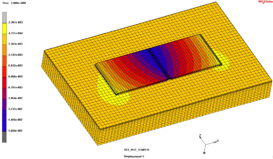
Рисунок 103 - Вертикальные перемещения плит покрытия от температурного воздействия и давления от колеса в углу плиты
