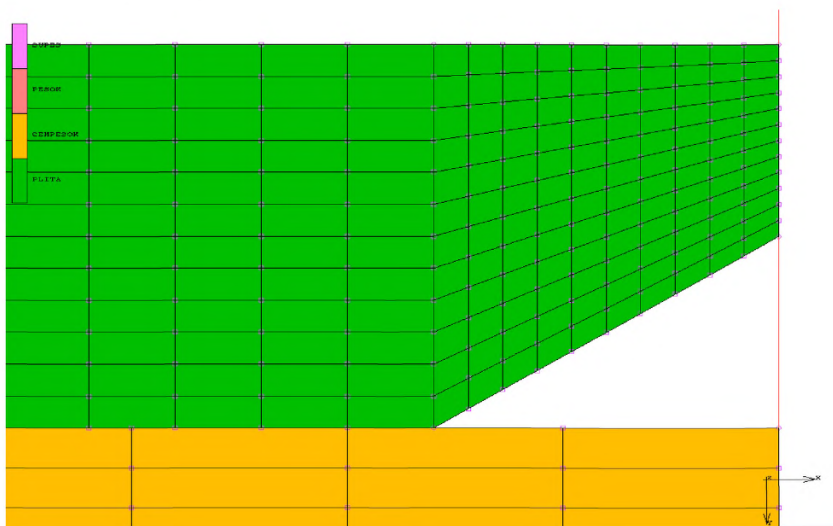
Рисунок 70– Конечно-элементная сетка в области поперечного шва
