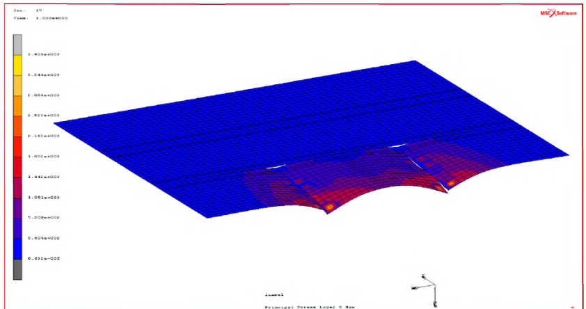
Рисунок 137–Распределение главных растягивающих напряжений \sigma_{\max} в верхнем слое жесткого автомобильно-дорожного покрытия
