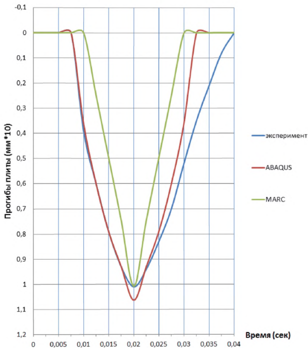
Рисунок 8 – Сравнение перемещений центральной точки верхней грани плиты в зависимости от времени, найденных в работе [18] и вычисленное с помощью КЭ комплекса «MARC-MENTAT».
