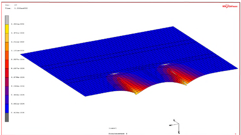
Рисунок 134–Вертикальные перемещения 3-полосного жесткого автомобильно-дорожного покрытия
