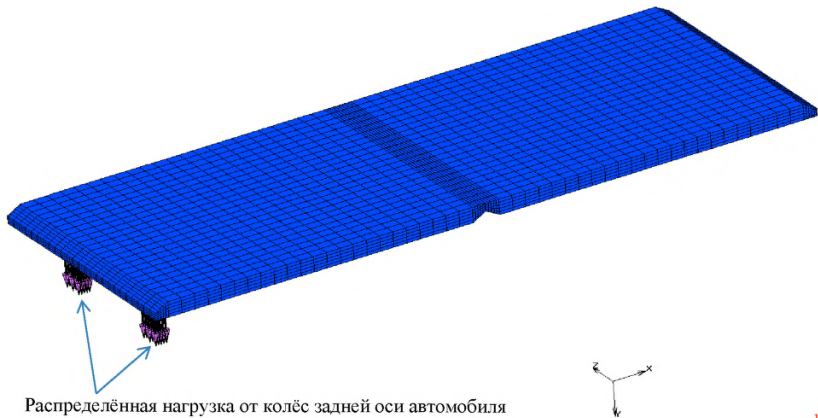
Распределённая нагрузка от колёс задней оси автомобиля
