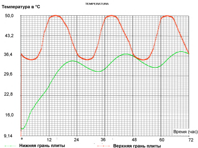
Рисунок 82– Изменение температуры на верхней и нижней гранях плиты в течении трёх суток
