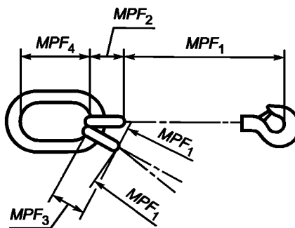
б) Стропальная цепь из двух жгутов
