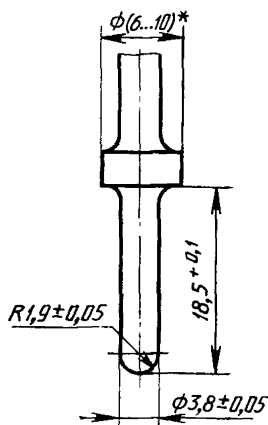
* Размер для справок. Черт. 15
