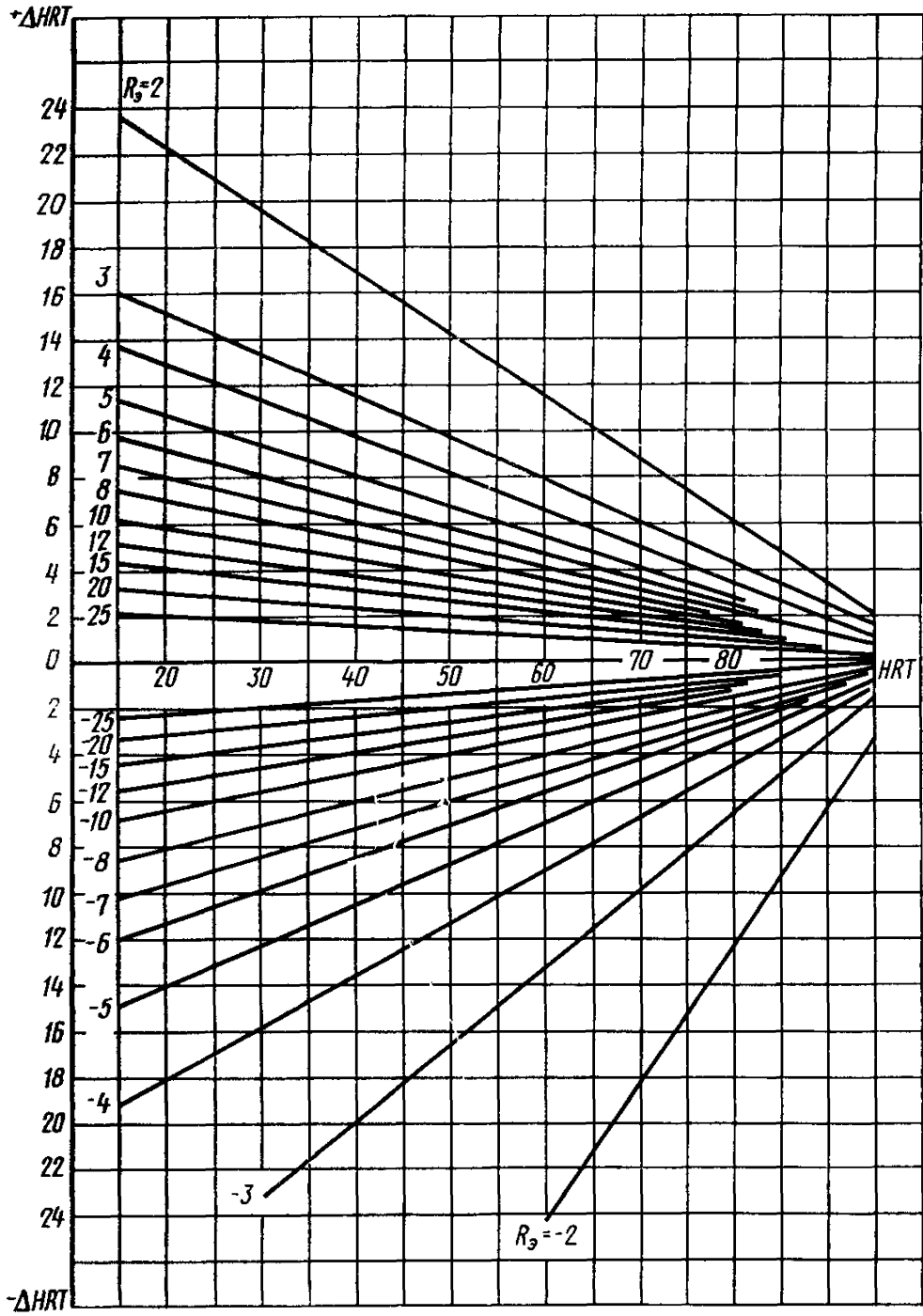
Черт 2
