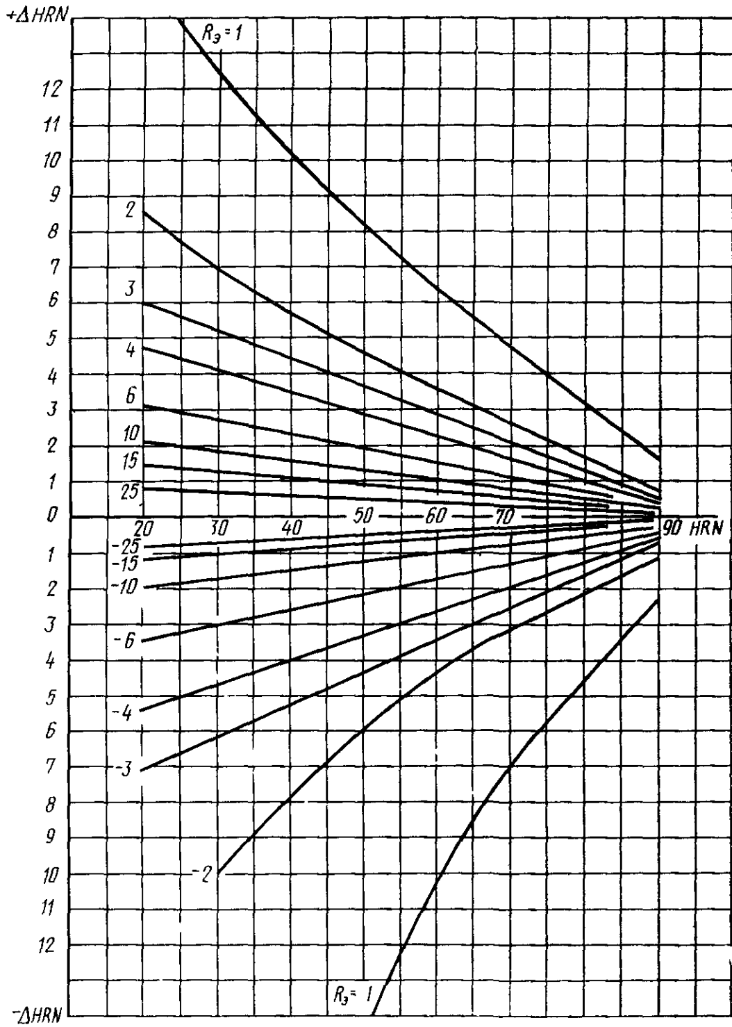
Черт. 1
