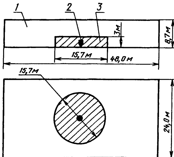
1 – помещение; 2 – аппарат; 3 – взрывоопасная зона
