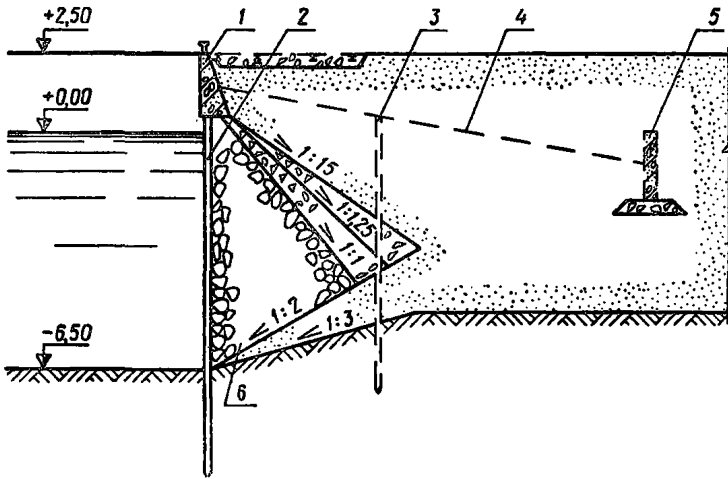
Рис. 1. Схема поперечного разреза причала типа больверк: 1—оголовок; 2—железобетонный шпунт; 3—деревянная свая; 4—анкерная тяга; 5—анкерная плита; 6—каменная призма
