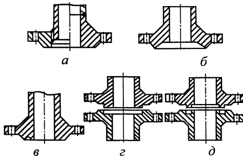
Рис. 1. Уплотнительные поверхности фланцев арматуры и соединительных частей трубопроводов: а – гладкая; б – под линзовую прокладку; в – под кольцевую прокладку овального сечения; г – выступ-впадина; д – шип-паз
